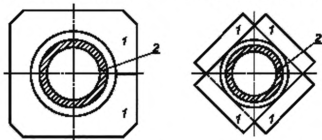
1 — сегментная катушка; 2 — труба
