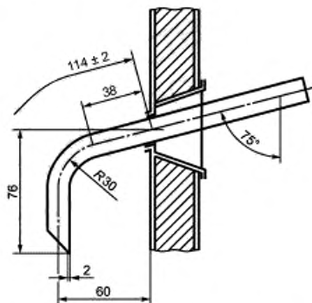
Рисунок А2.3 — Нижний конец трубки холодильника
