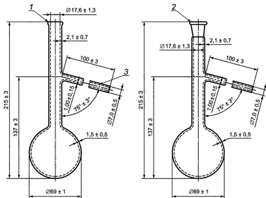
1 — усиливающий валик; 2 — муфта 19/22 или 19/26; 3 — огневая полировка стекла
