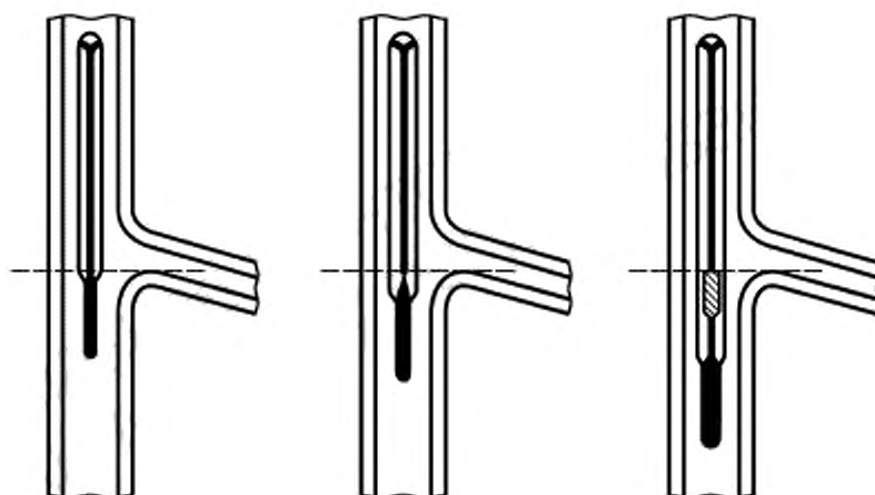
Рисунок 5 — Положение термометра в перегонной колбе
