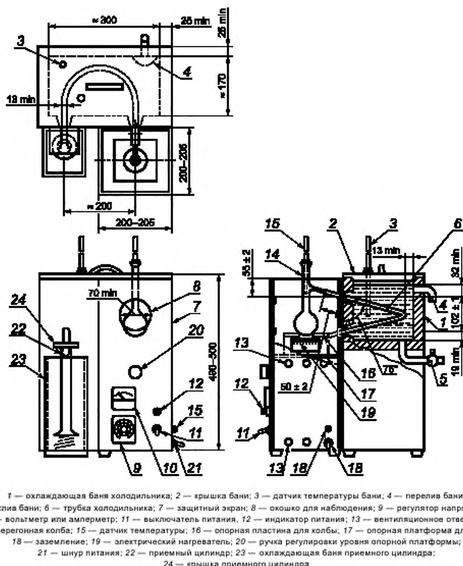
Рисунок 2 — Аппарат в сборе с электрическим нагревателем
