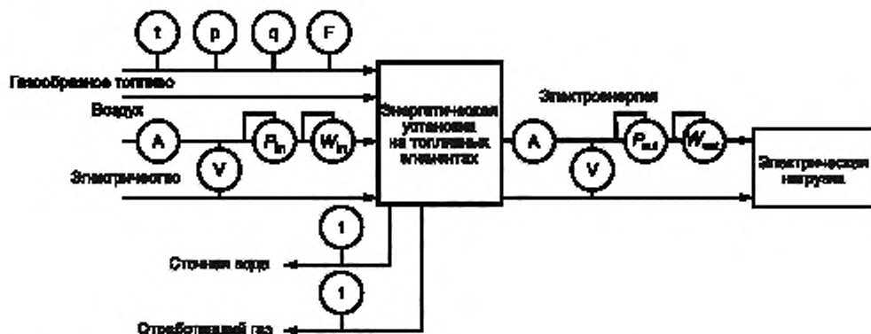
А — амперметр; В — вольтметр; t — термометр; p — манометр; q — расходомер; F — интегрирующий расходомер; P — ваттметр; W — интегрирующий ваттметр (электрический счетчик); сточная вода — для измерения объема (или массы); рН, БПК, ХПК; отработавший газ — к общему устройству для анализа компонентов
