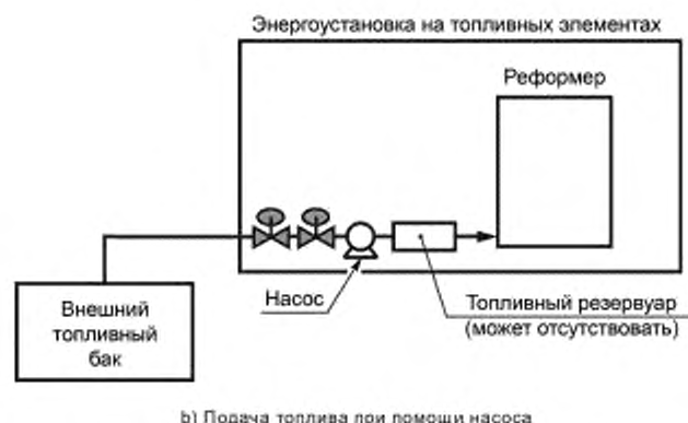
Рисунок 9 — Примеры систем подачи жидкого топлива
