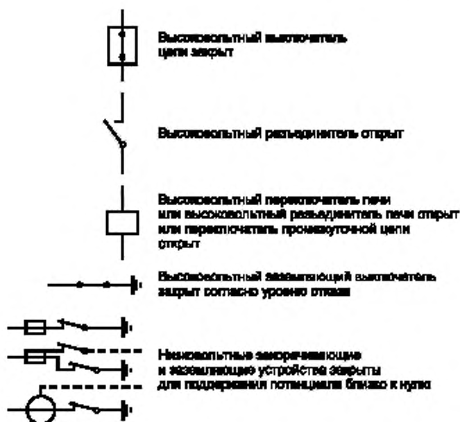
Рисунок АА.5 — Источник постоянного тока печи с высоковольтным переключателем (или высоковольтным выключателем печи) в закрытом положении, клапанные импульсы запуска остановлены, и переключатель низковольтного разъединителя в открытом положении
