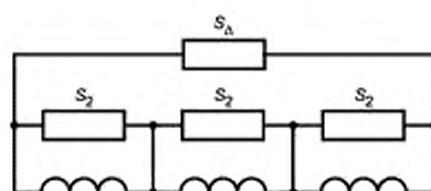
Рисунок 1 — Схема подключения фазных нагрузок
