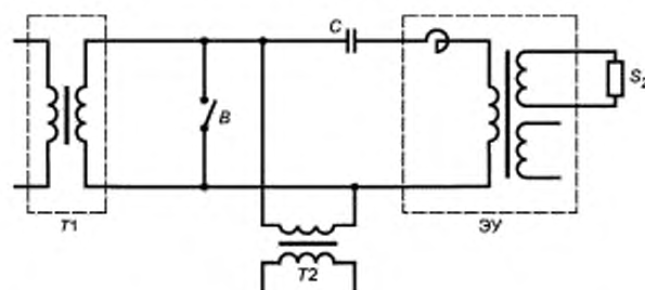
T1 — питающий трансформатор; C — конденсатор отбора мощности емкостного трансформатора; T2 — трансформатор напряжения для осциллографирования; ZY — электромагнитное устройство емкостного трансформатора; B — высоковольтный короткозамыкатель; S2 — нагрузка основной вторичной обмотки
