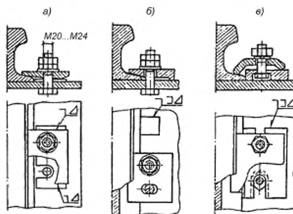
а) планка упорная расположена под прижимной планкой без сварки с подкрановой балкой; б) планка упорная расположена вне прижимной и сварена с подкрановой балкой; в) планка упорная расположена под прижимной и сварена с подкрановой балкой. Данная конструкция крепления не требует создания отверстий в подкрановой балке под крепежные болты.
