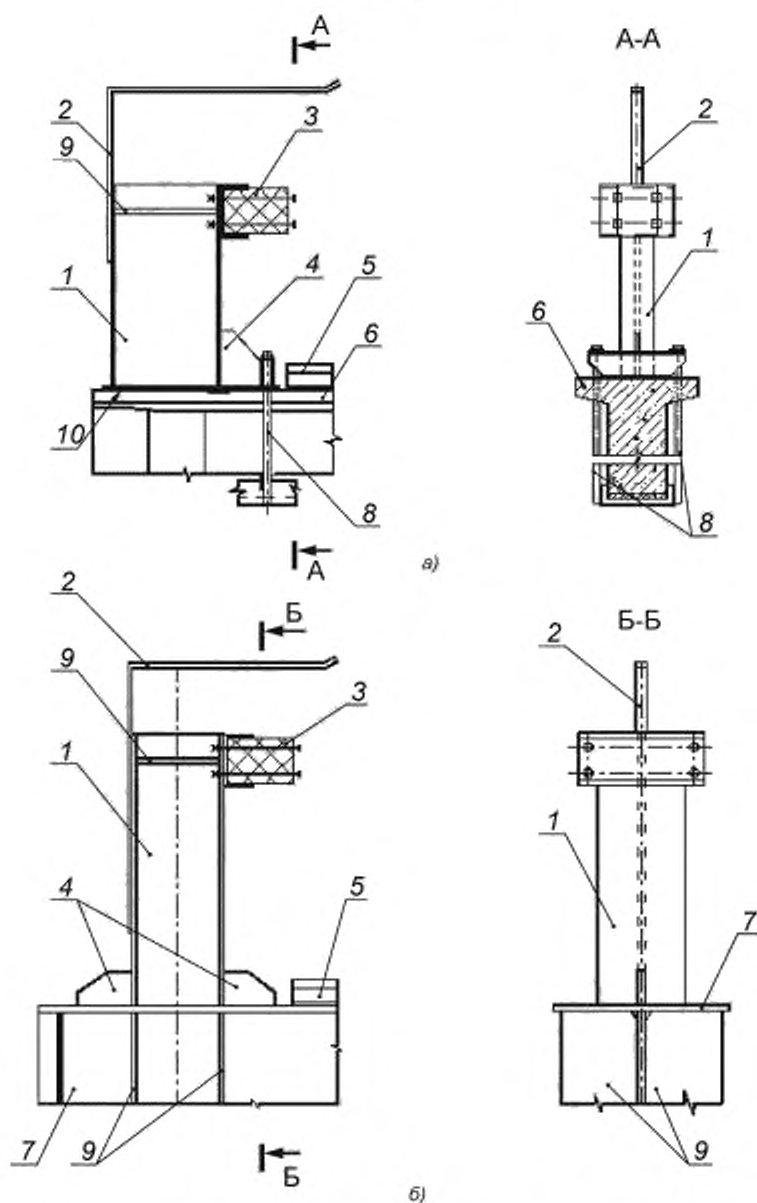
Рисунок В.1 — Тупиковый упор ударного типа на железобетонной (а) и металлической (б) балке кранового пути
