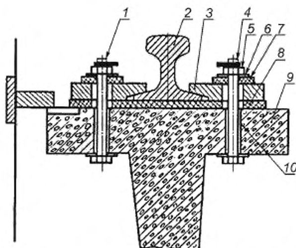
1 — болт, 2 — рельс, 3 — планка прижимная, 4 — стопорная шпилька, 5 — гайка, 6 — шайба, 7 — упругая прорезиненная прокладка, 8 — упругая прорезиненная лента, 9 — бетонная подкрановая балка, 10 — металлическая труба
