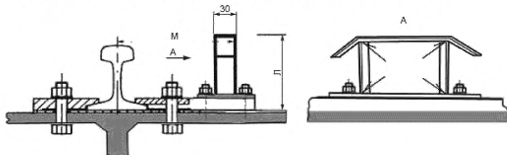
Рисунок В.3 — Типовая конструкция отключающей линейки
