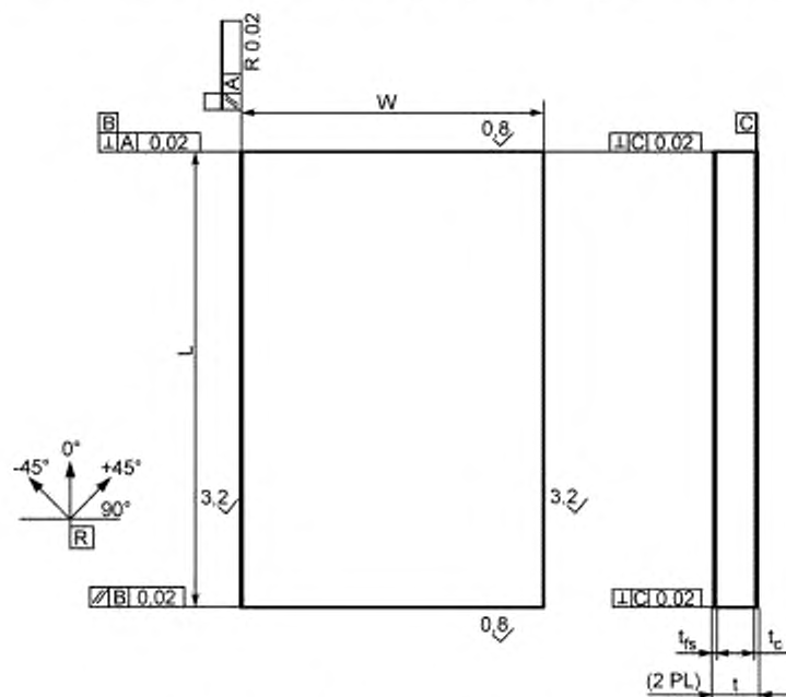
Рисунок 1 — Размеры образцов
