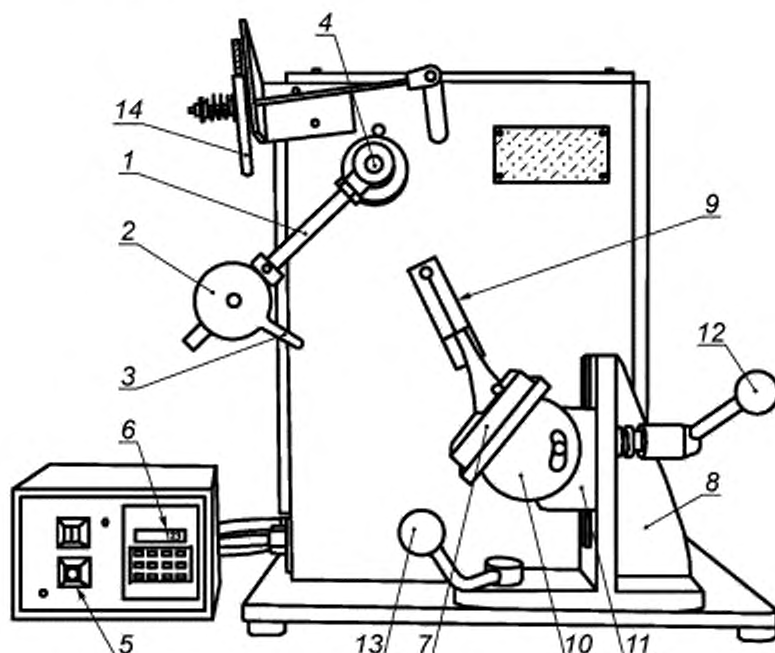
1 — маятник; 2 — груз маятника; 3 — головка бойка; 4 — стулица; 5 — выключатель электрического питания; 6 — счетчик; 7 — держатель образца для испытаний; 8 — вертикальная установочная плита; 9 — направляющая пластина, используемая при установке каблук; 10 — основной зажим для ориентации вращения; 11 — зажим для вертикальной ориентации; 12 — устройство для регулировки расположения зажимов 10 и 11 относительно вертикальной установочной плиты 8; 13 — устройство для регулировки в горизонтальной плоскости; 14 — амортизатор обратного хода
