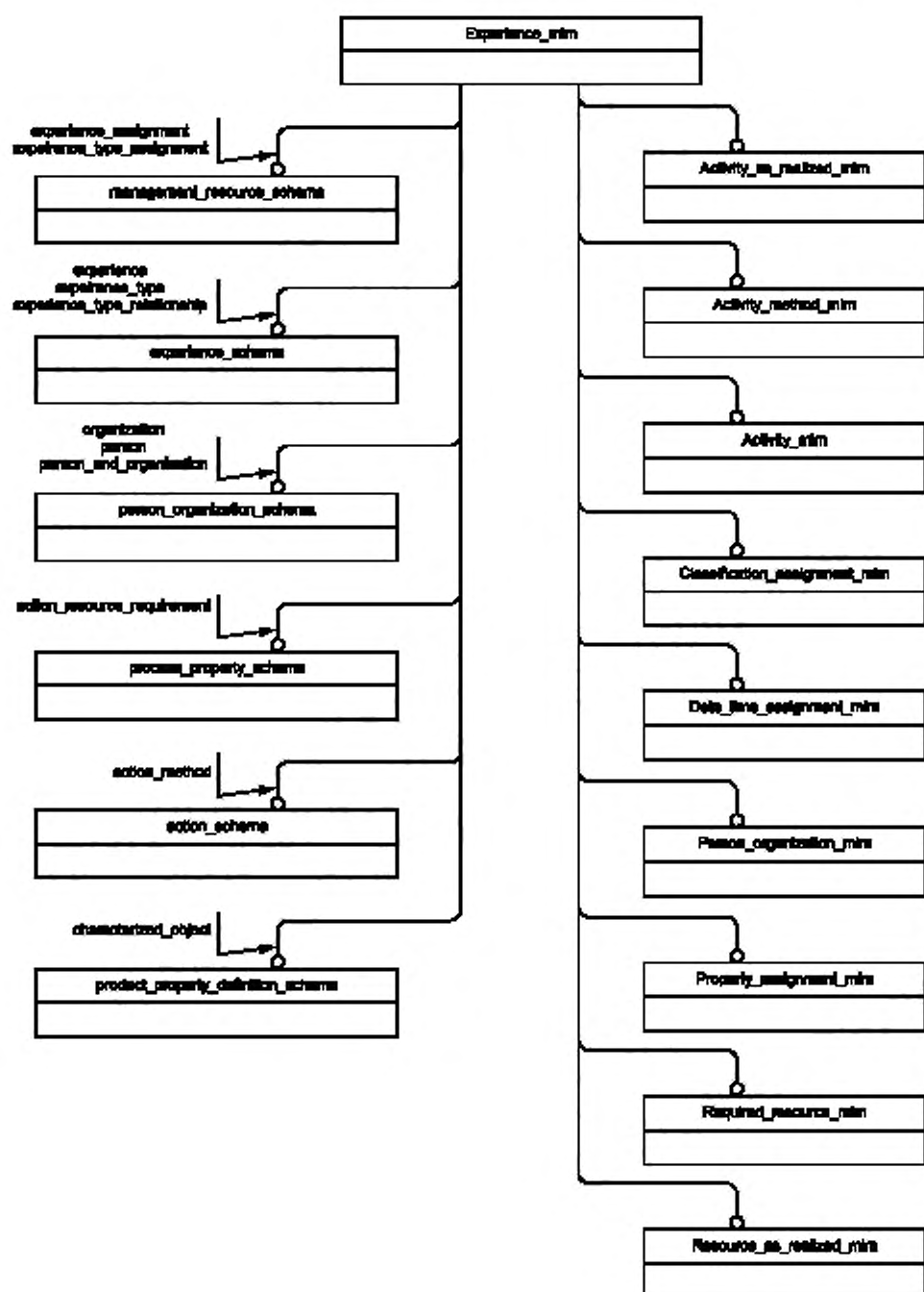
Рисунок D.1 — Представление IMM на уровне схем в формате EXPRESS-G (диаграмма 1 из 1)
