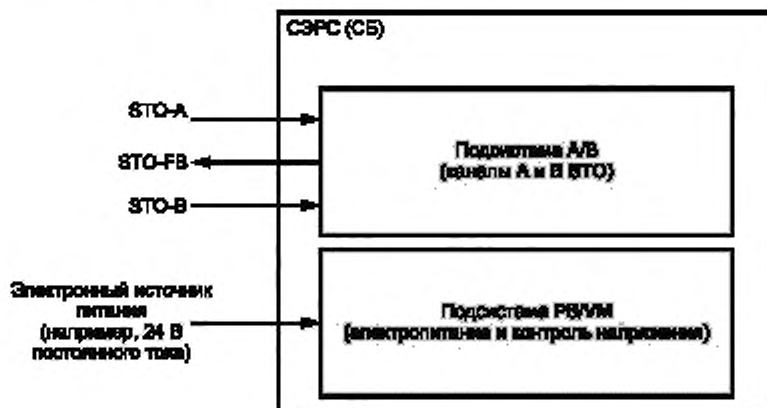
Рисунок В.2 — Подсистемы СЭРС (СБ)
