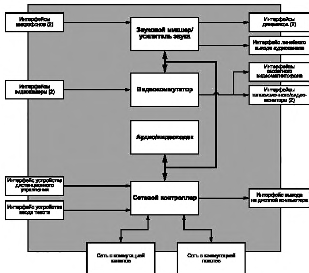
Рисунок 11 — Содержание коммуникационного контроллера связи системы учащегося
