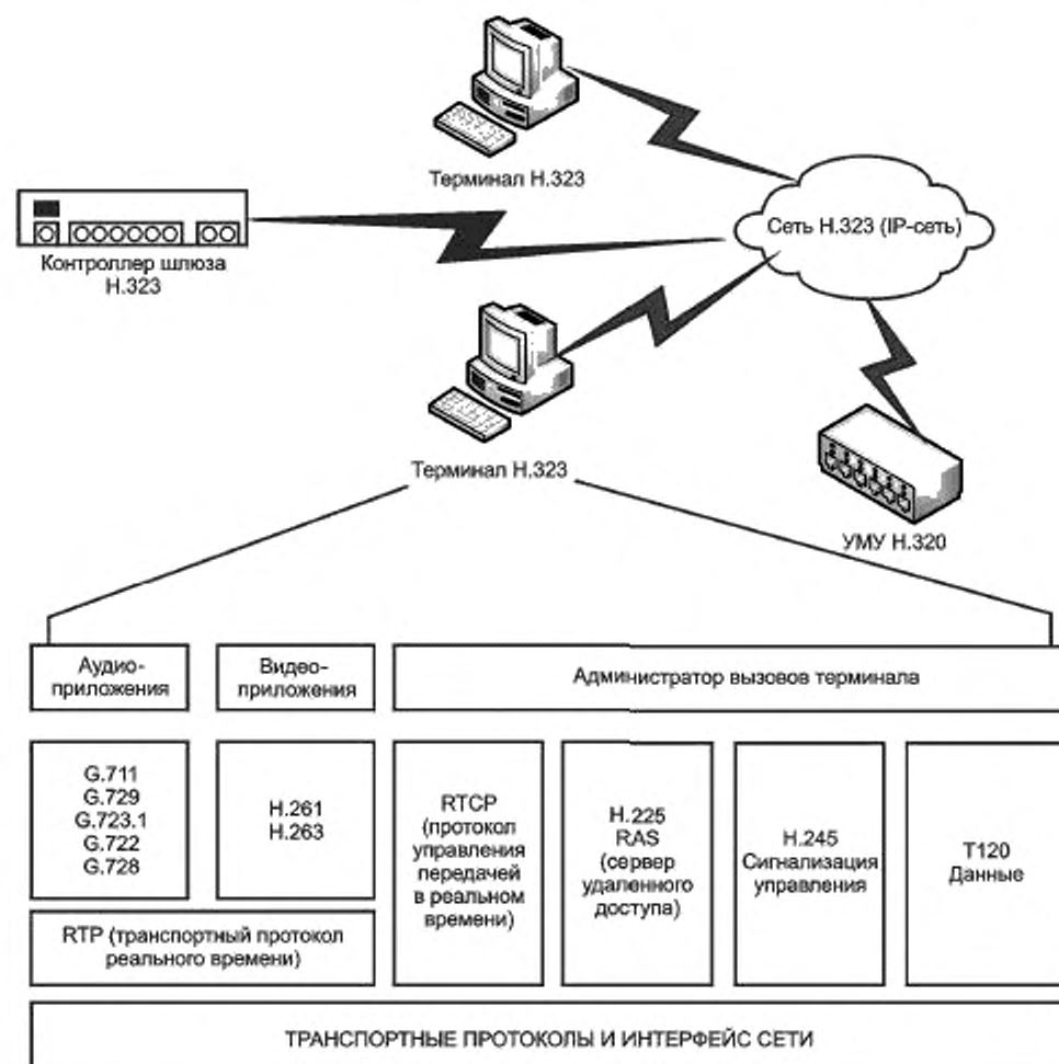
Рисунок 13 — Интероперабельность H.323
