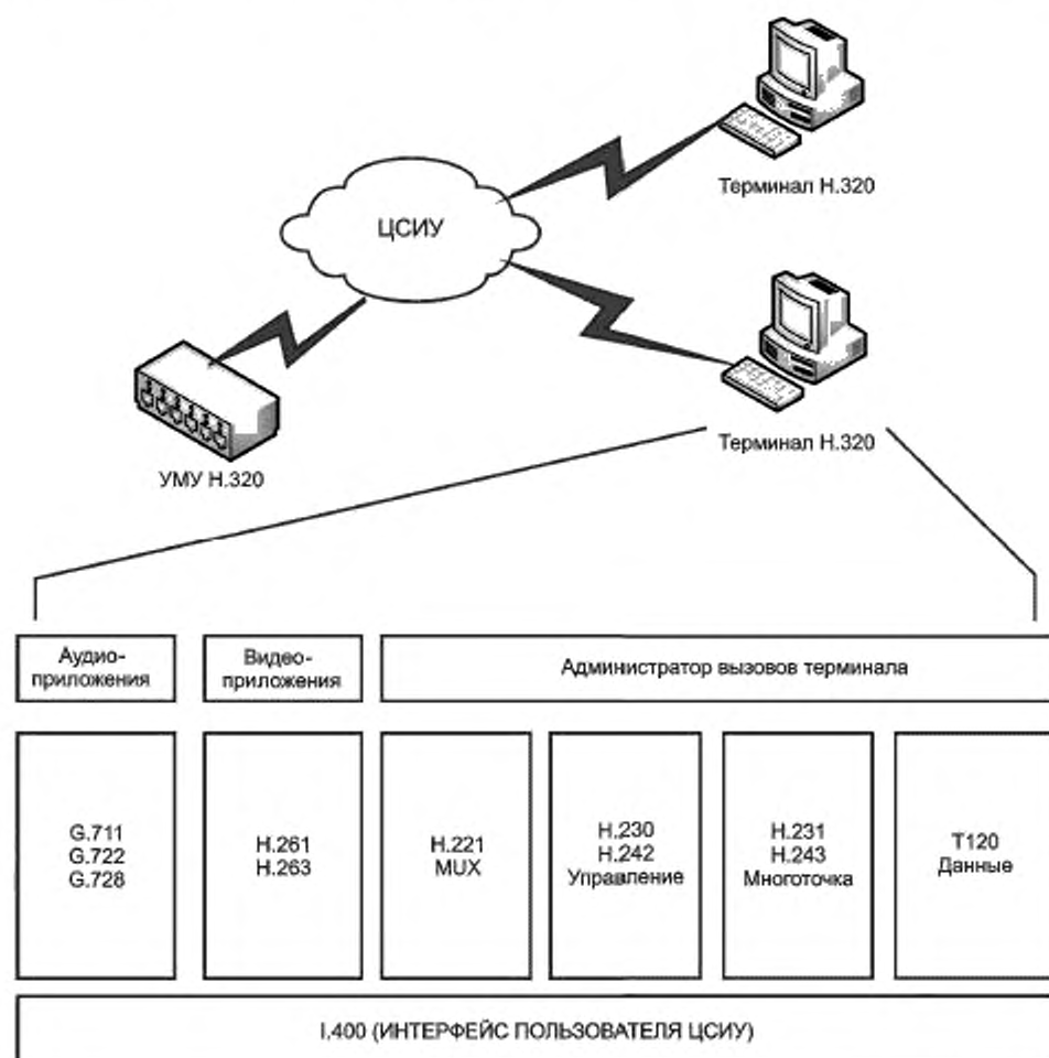
Рисунок 12 — Интероперабельность H.320
