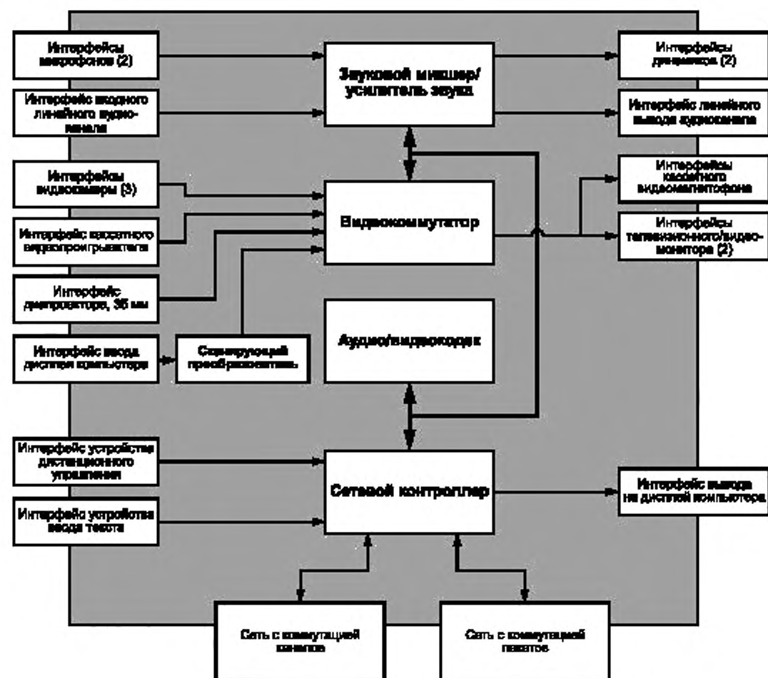
Рисунок 9 — Содержание коммуникационного контроллера системы инструктора
