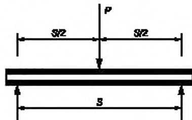
(a) трехточечное нагружение (C393/C393M стандартная схема)
