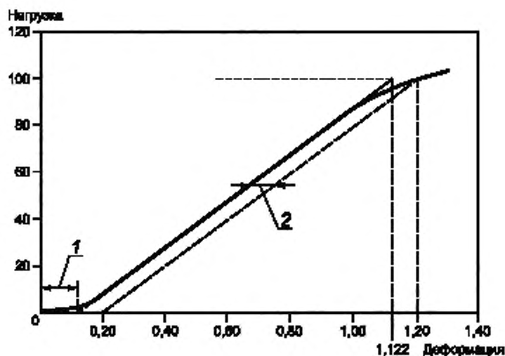
1 — поправка на изначальную нелинейность; 2 — отклонение от линейности
