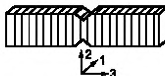
Рисунок 3 — Ориентация слоев в образцах для определения свойств при сдвиге в шести различных направлениях
