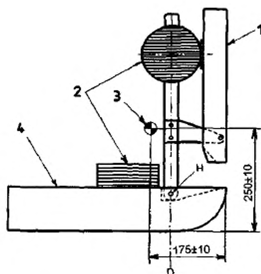
Рисунок А.3 — ЭНУВ — Положение центра тяжести
