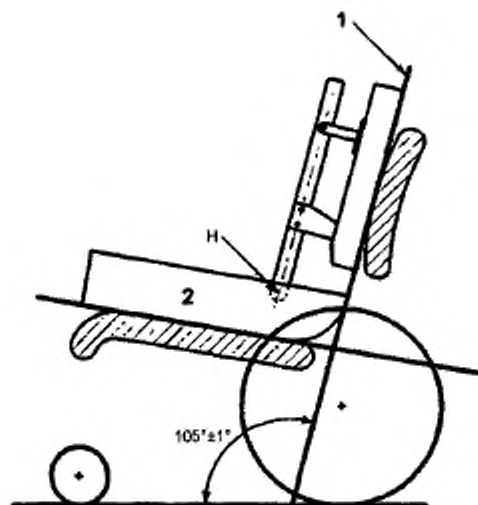
1 — базовая плоскость спинки; 2 — ЭНУ
