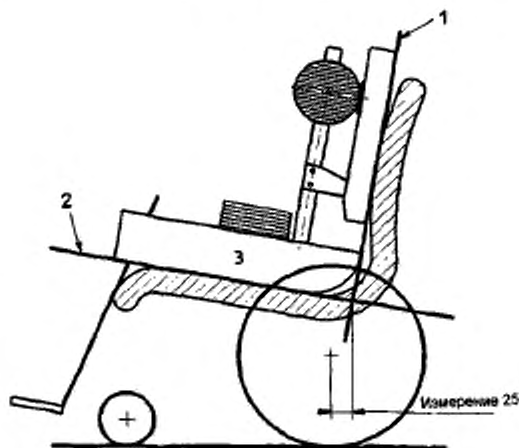
а) Горизонтальное положение оси ведущего колеса
