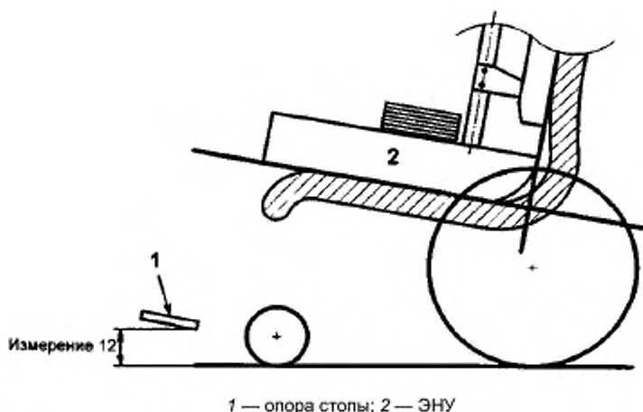
Рисунок 21 — Клиренс опоры стопы
