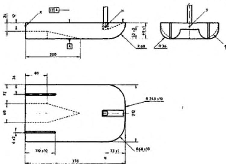
Рисунок А.4 — Узел сиденья ЭНУВ
