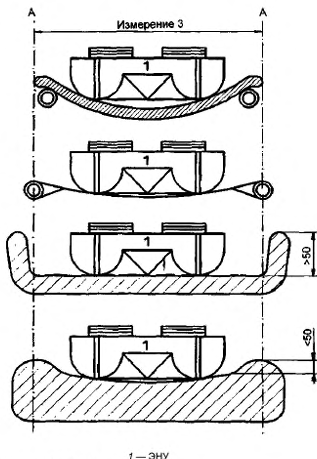
1 — ЭНУ b) Ширина сидений для различных типов сидений
