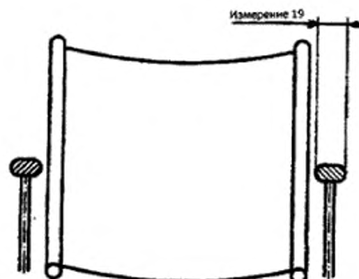
Рисунок 28 — Ширина подлокотника
