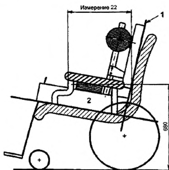
Рисунок 31 — Расположение подлокотника
