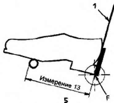
d) Длина опоры стопы трубчатой формы с задником-держателем
