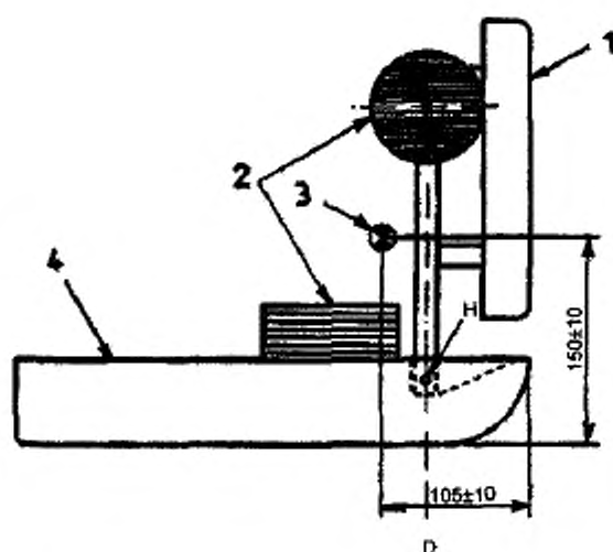
Рисунок А.6 — Положение центра тяжести ЭНУР
