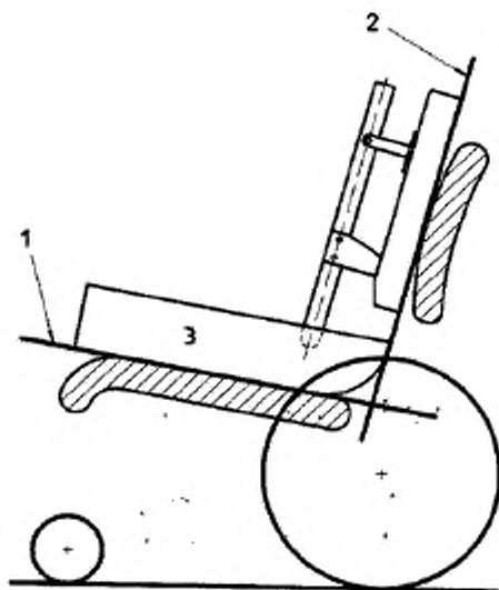
1 — базовая плоскость сиденья; 2 — базовая плоскость спинки; 3 — ЭНУ
