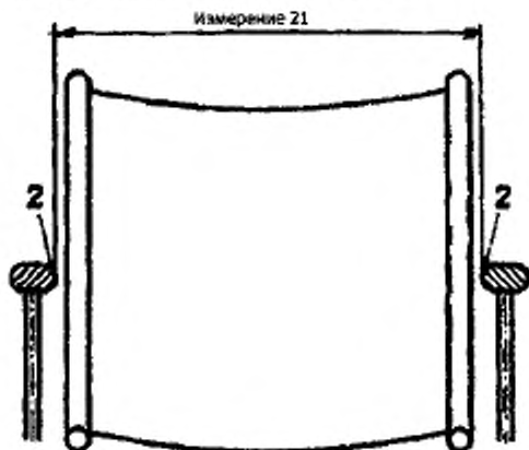
Рисунок 30 — Расстояние между подлокотниками
