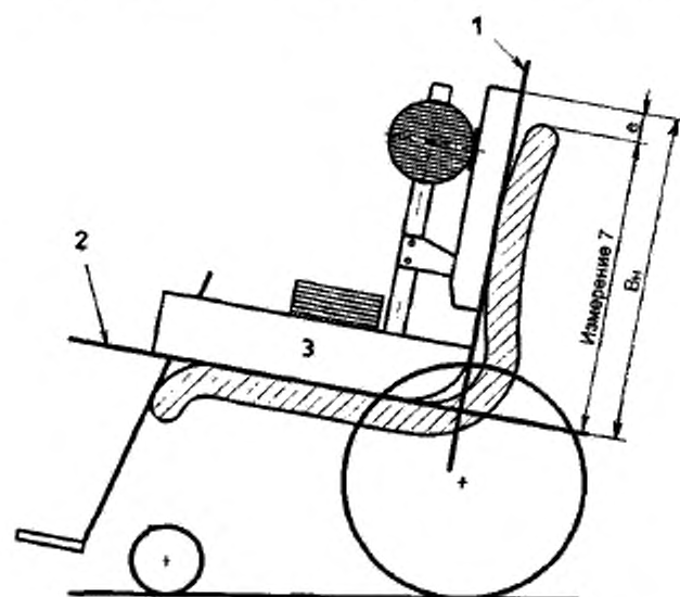
1 — базовая плоскость спинки; 2 — базовая плоскость сиденья; 3 — ЭНУ
