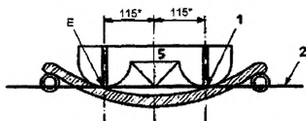
Рисунок 20 — Длина подножки
