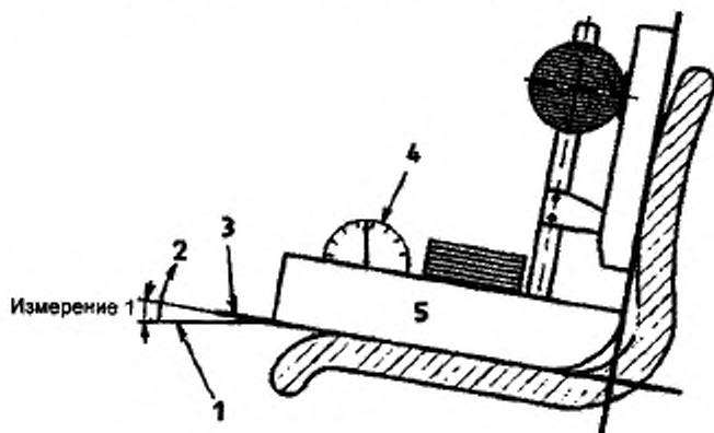
1 — горизонталь; 2 — положительное направление; 3 — базовая плоскость сиденья;
