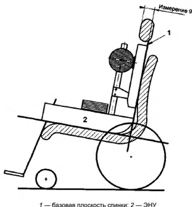
Рисунок 18 — Подголовник впереди спинки
