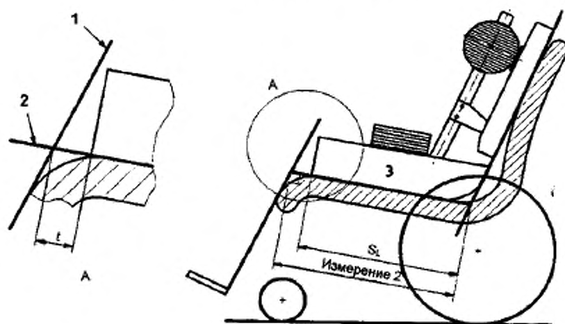
Рисунок 11 — Глубина сиденья
