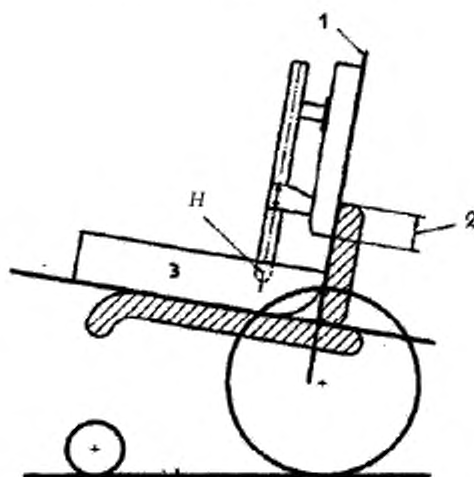
1 — базовая плоскость спинки;
