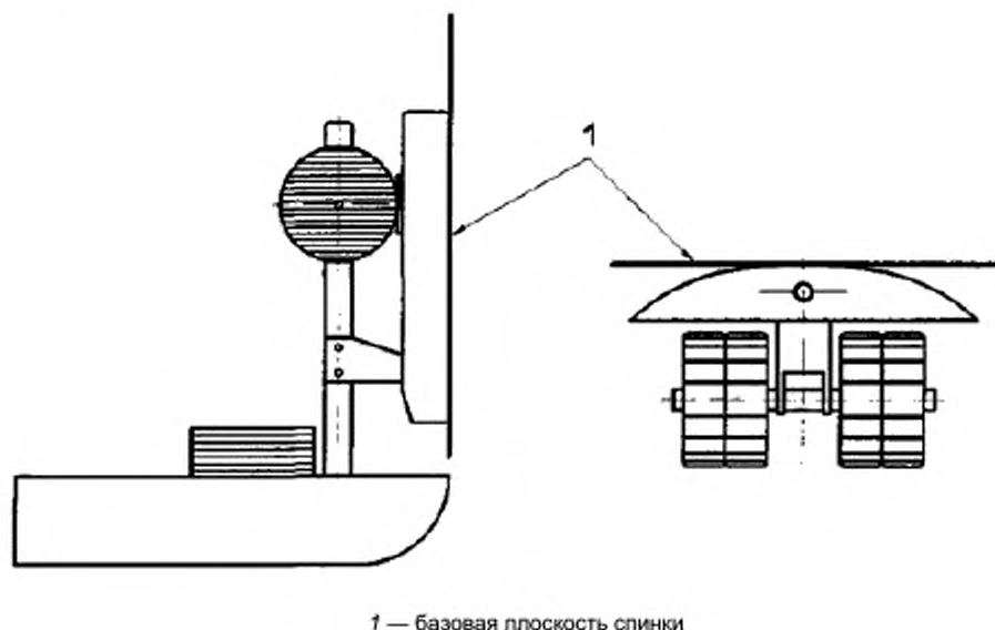
Рисунок 2 — Базовая плоскость спинки
