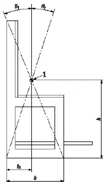
Рисунок А.3 — Рассчитываемые величины для метода балансировки
