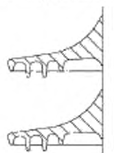
Рисунок 5 — Типичный профиль с глубокими канавками под ребром
