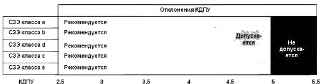
Рисунок 16 — Рекомендации по выбору коэффициента длины пути утечки
