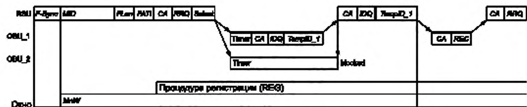
Рисунок 13 — Регистрационная процедура без столкновения
