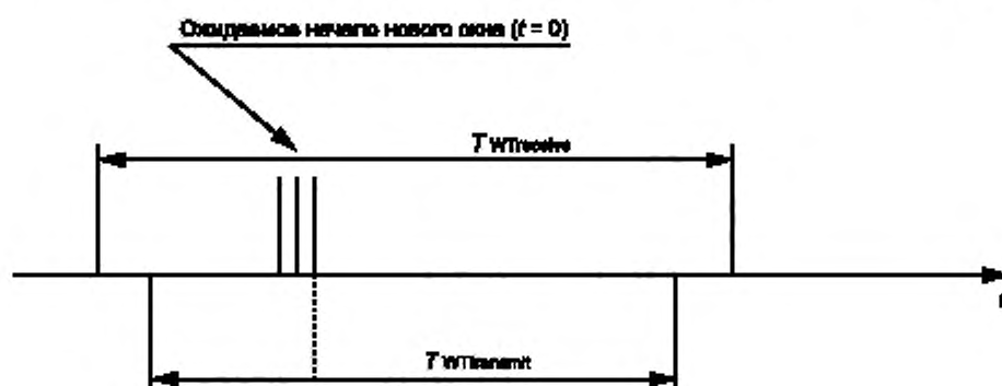
Рисунок 8 — Окно синхронизации (W-Sync) приемника и окно передатчика
