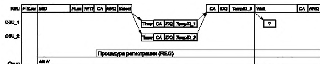
Рисунок 14 — Регистрационная процедура со столкновением
