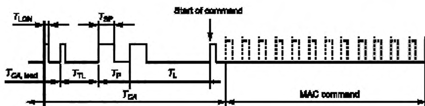
Рисунок 12 — Команда внимание (CA)
