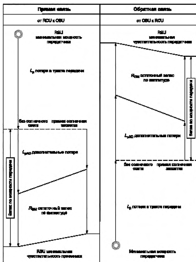
Рисунок С.1 — Схема бюджета питания связи
