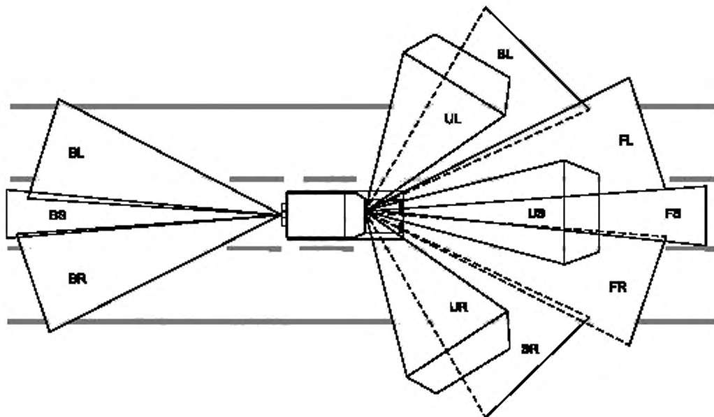
Рисунок D.3 — Коммуникационные зоны, вид сверху
