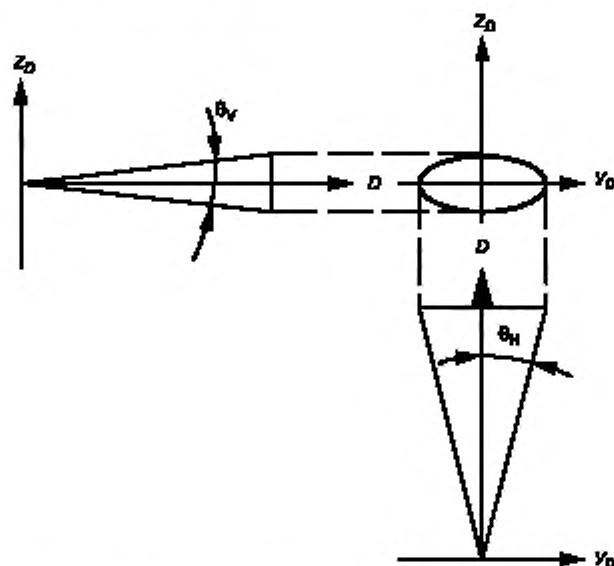
Рисунок 5 — Открытые горизонтальный и вертикальный углы
