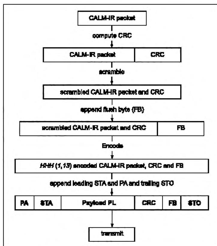
Рисунок В.1 — CALM-fast IR обработка пакета
