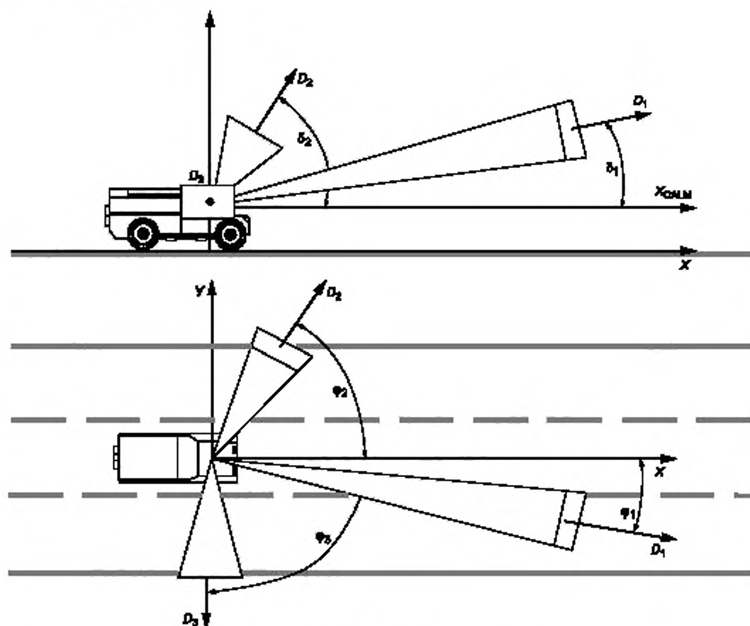
Рисунок D.1 — Многолучевая антенна
