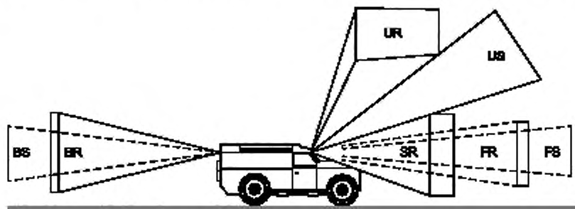
Рисунок D.2 — Вид сбоку коммуникационных зон
