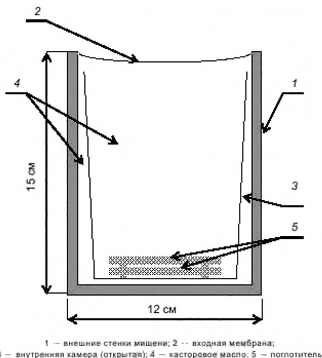
Рисунок D.1 — Схема расширяющейся мишени
