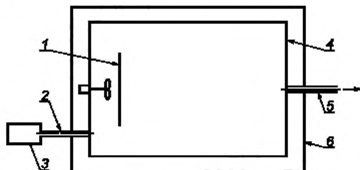
1 — циркуляция воздуха; 2 — контролируемый увлажненный поток; 3 — система подачи чистого воздуха; 4 — небольшая камера; 5 — линия отбора проб; 6 — термостатированная испытательная камера
