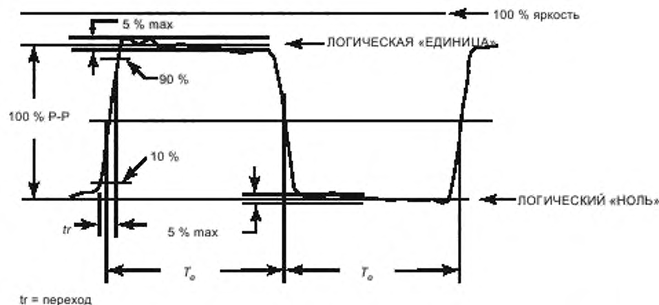
Рисунок 8 — Форма волны вертикального интервального (полевого) временного кода
