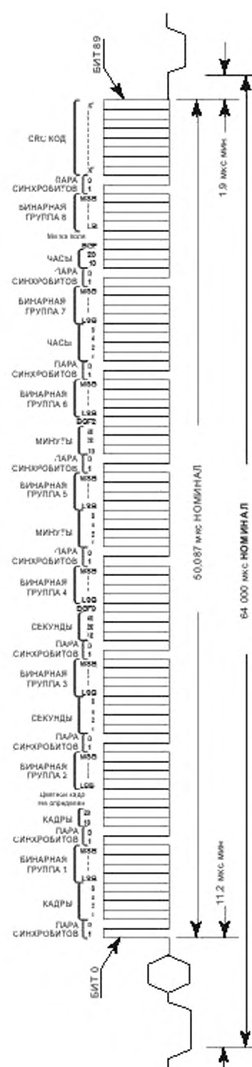
Рисунок 7 — Распределение и синхронизация адресного бита вертикального интервала (полевого) временного кода для режима 625/50
