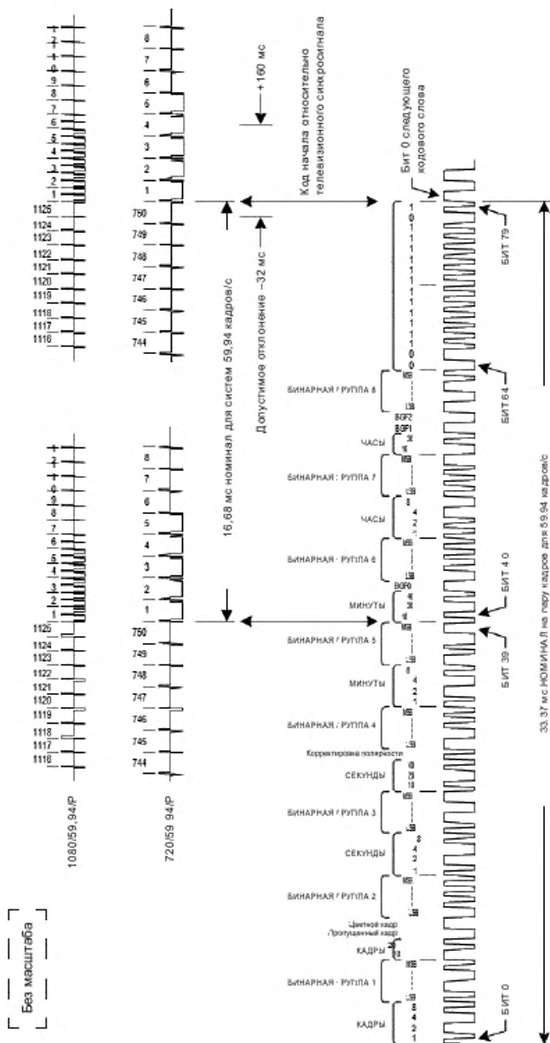
Рисунок 5 — Пример линейного временного кода по отношению к 59,94-кадровому последовательному видеосигналу
