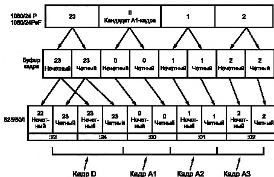
Рисунок В.2 — Пример преобразования видеосигнала высокой четкости с частотой 24 кадр/с в видеосигнал 625/50/строка
