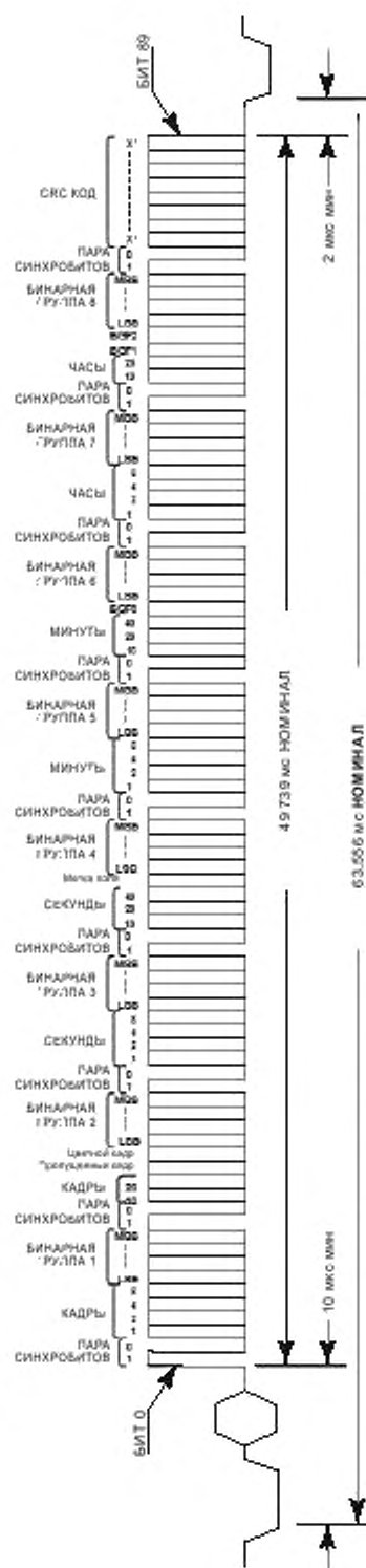
Рисунок 6 — Распределение и синхронизация адресного бита вертикального интервала (полевого) временного кода для режима 525/59.94
