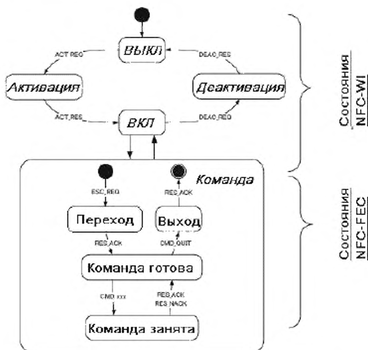
Рисунок 1 — Состояния NFC-WI и подсостояния NFC-FEC
