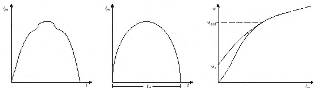
Рисунок 2B.14 — Осциллограммы, зарегистрированные при использовании метода разрядки конденсатора
