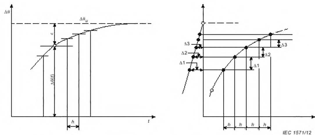
Рисунок 2D.1 — Графическая экстраполяция к окончательному превышению температуры
