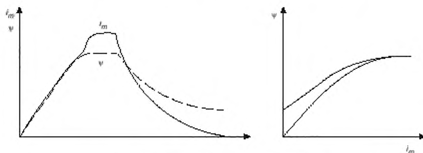
Рисунок 2B.11 — Диаграмма потоков и токов насыщения
