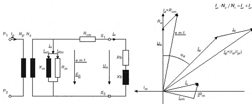
Рисунок 2Е.1 — Упрощенная эквивалентная цепь трансформатора тока
