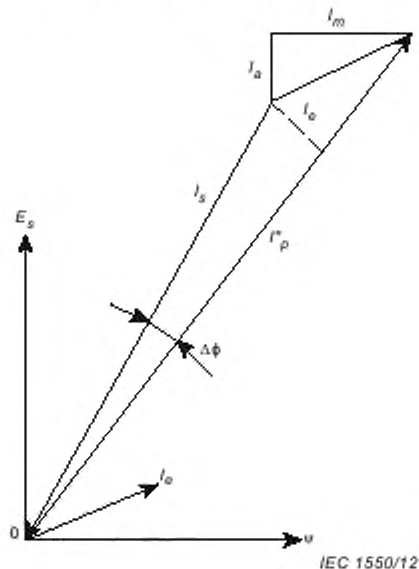
Рисунок 2А.1 — Векторная диаграмма
