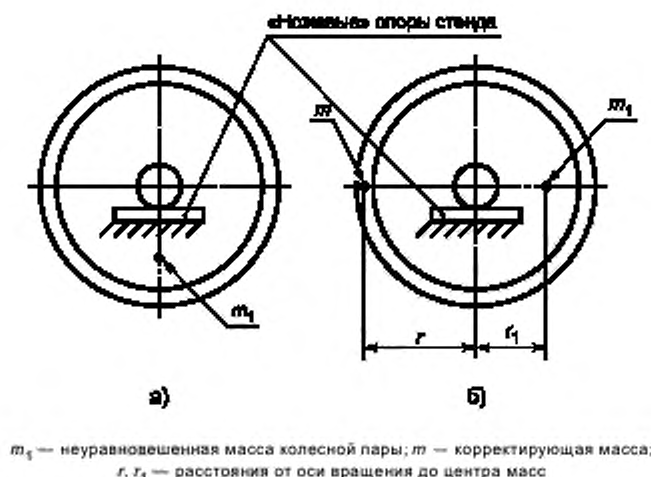
Рисунок 2 — Схема статического уравнивания колесной пары
