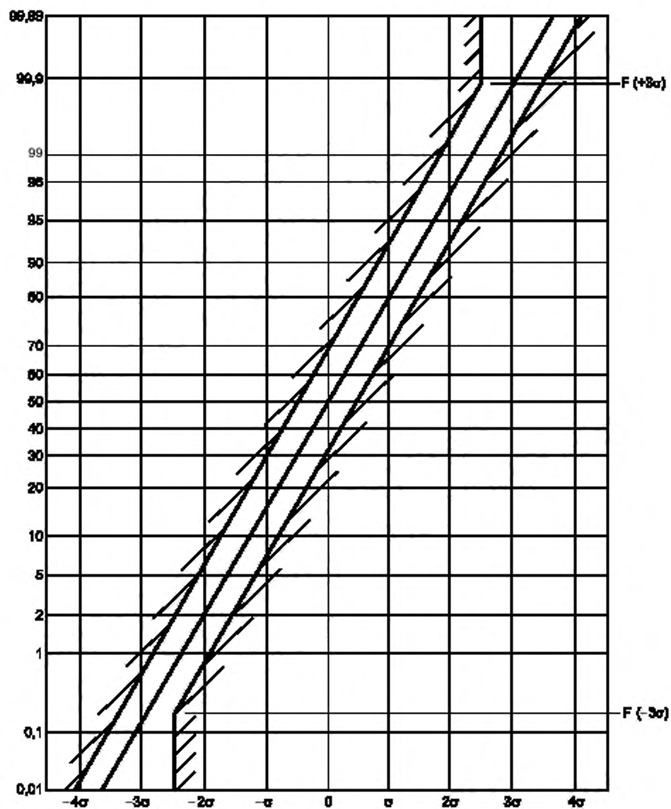
Рисунок 5 — Поля допуска для интегральной плотности распределения вероятности
