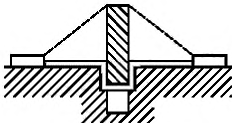
Рисунок E.8 — Расстояние утечки на примере 7
