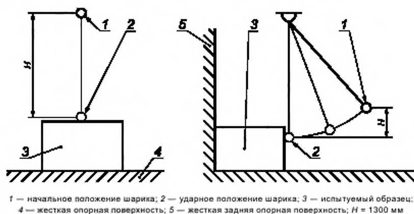
Рисунок 8 — Устройство для механических испытаний на устойчивость к механическим ударам (9.2.6.2.1)
