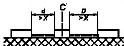
Рисунок E.11 — Расстояние утечки на примере 10
