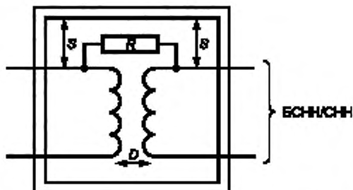
Рисунок 1.1 — Пример подсоединения защитного сопротивления между разделенными цепями
