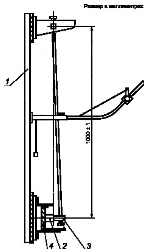
1 — рама; 2 — образец; 3 — ударный элемент; 4 — монтажная опора
