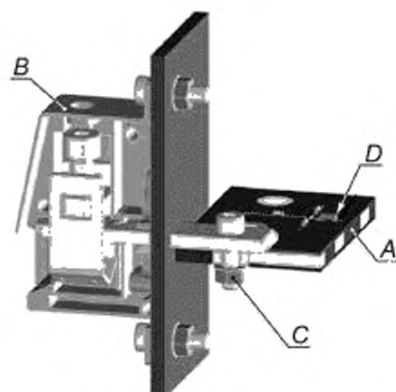
A — печатная плата; B — клеммная колодка для монтажа на печатной плате, C — подключение по 7.1.2; D — компонент SMD (устройство для поверхностного монтажа)
