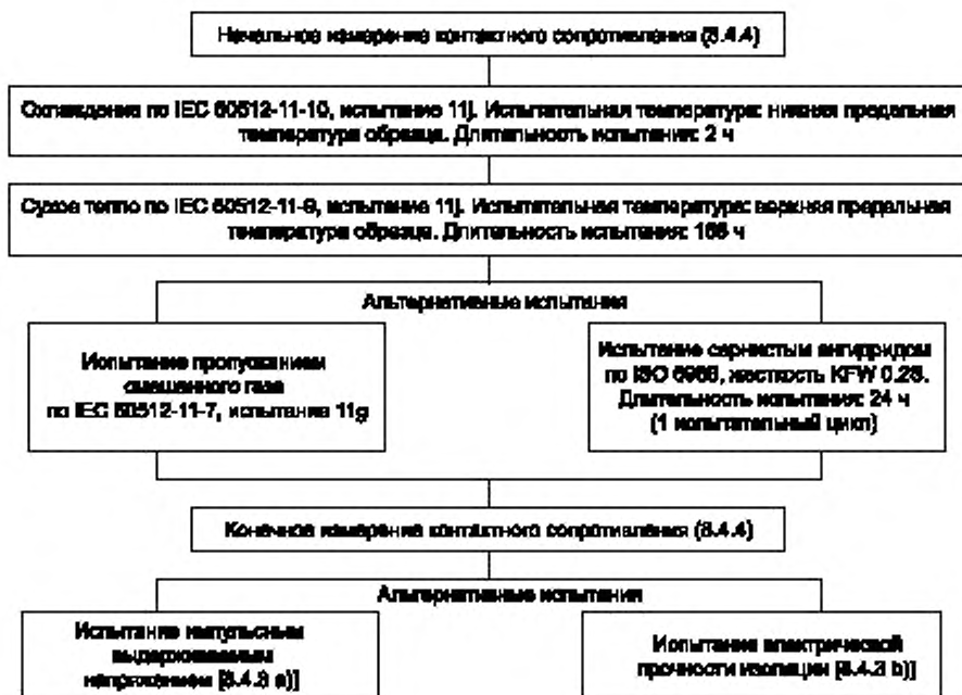
Рисунок 4 — Последовательность испытания
