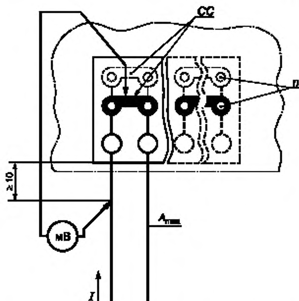
Рисунок 3 — Испытательное устройство для измерения кратковременно допустимого тока
