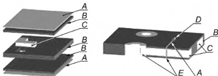
Рисунок С.1 — Структура печатной платы на большие токи
