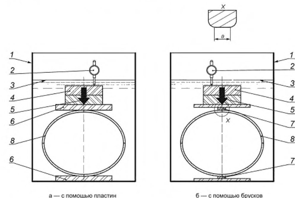
1 — емкость с водой; 2 — датчик деформации; 3 — уровень воды; 4 — статическая нагрузка; 5 — сжимающая нагрузка F ; 6 — пластины; 7 — бруски; 8 — образец для испытаний; а — ширина плоской поверхности бруска
