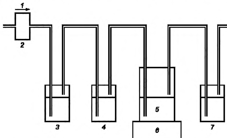
1 — сжатый воздух; 2 — расходомер; 3 — ловушка диоксида углерода ( \text{NaOH} ); 4 — индикатор диоксида углерода [ \text{Ba}(\text{OH})_2 ]; 5 — испытательные сосуды; 6 — мешалка; 7 — ловушка диоксида углерода [ \text{Ba}(\text{OH})_2 или ( \text{NaOH} )]
