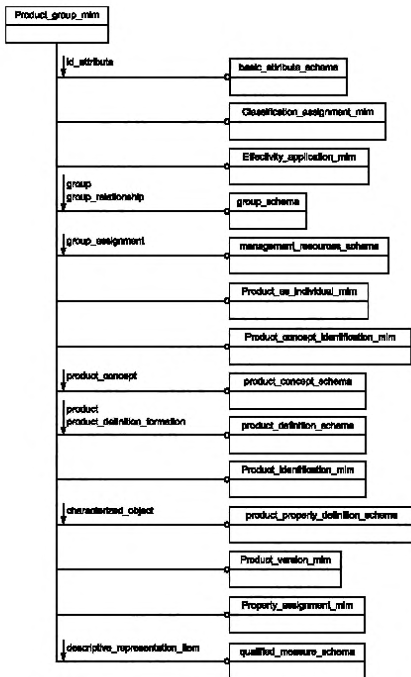
Рисунок D.1 — Представление IMM на уровне схем в формате EXPRESS-G
