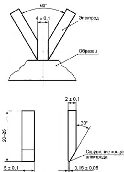
Рисунок 9 — Расположение и размеры электродов для испытания на трекинговость
