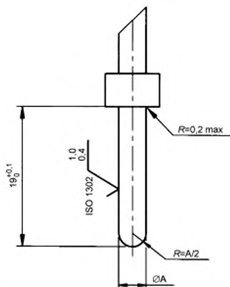
Рисунок 4 — Система вилок и штепсельных розеток на 16 А, 250 В переменного тока. Калибр для проверки позиции 7 стандартных листов 1-1, 3-1 и 3-2
