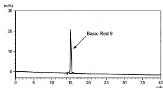
Рисунок А.2 — Хромотограмма ВЭЖХ/ДМД (основный красный 9), детектирование при длине волны 540 нм
