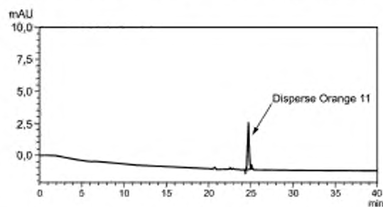
Рисунок А.4 — Хромотограмма ВЭЖХ/ДМД (дисперсный оранжевый 11), детектирование при длине волны 480 нм
