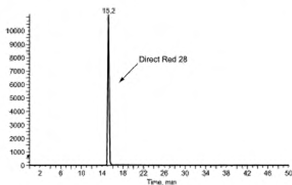
Рисунок А.42 — SRM-хроматограмма конго красного 28
