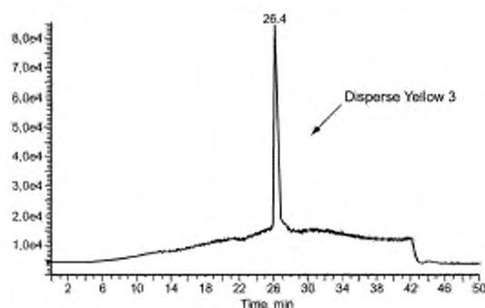
Рисунок А.20 — SIM-хроматограмма дисперсного желтого 3
