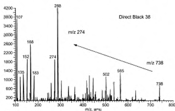
Рисунок А.39 — Масс-спектр дочерних ионов прямого черного 38
