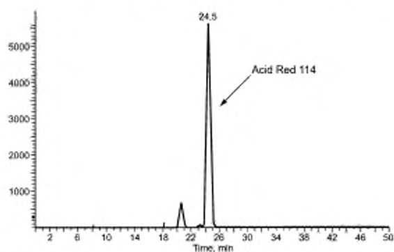
Рисунок А.36 — SRM-хроматограмма кислотного красного 114
