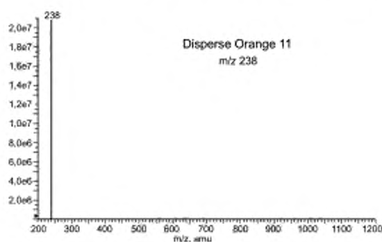
Рисунок А.17 — Масс-спектр дисперсного оранжевого 11
