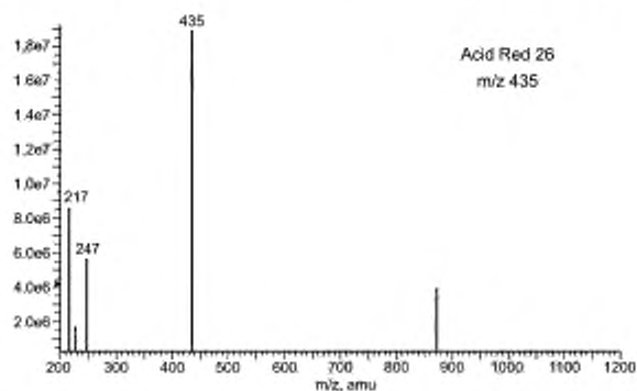
Рисунок А.23 — Масс-спектр кислотного красного 26
