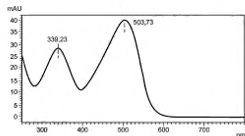
Рисунок А.13 — УФ-спектр конго красного 28
