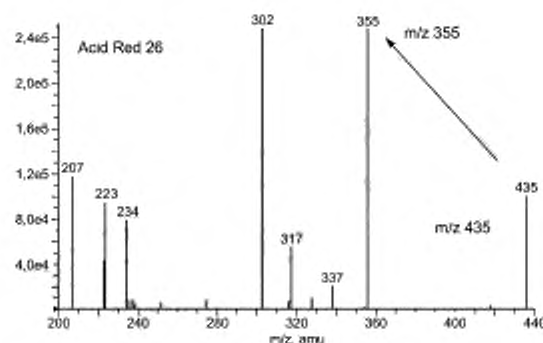
Рисунок А.37 — Масс-спектр дочерних ионов кислотного красного 26
