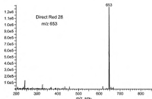
Рисунок А.27 — Масс-спектр конго красного 28
