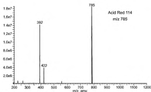
Рисунок А.21 — Масс-спектр кислотного красного 114
