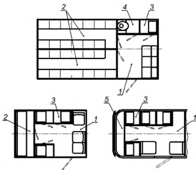
1 — помещение конвоя; 2 — общая камера(ы); 3 — одиночная камера(ы); 4 — туалетная кабина; 5 — вспомогательный отсек
