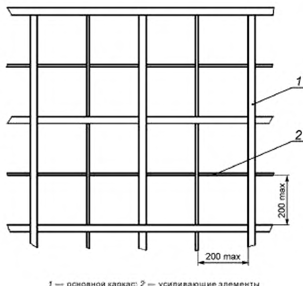
1 — основной каркас; 2 — усиливающие элементы
