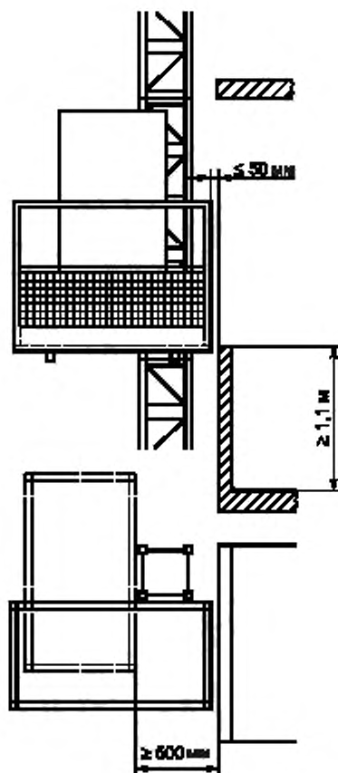
Рисунок 7 — Пример погрузочной площадки с неподвижным защитным устройством
