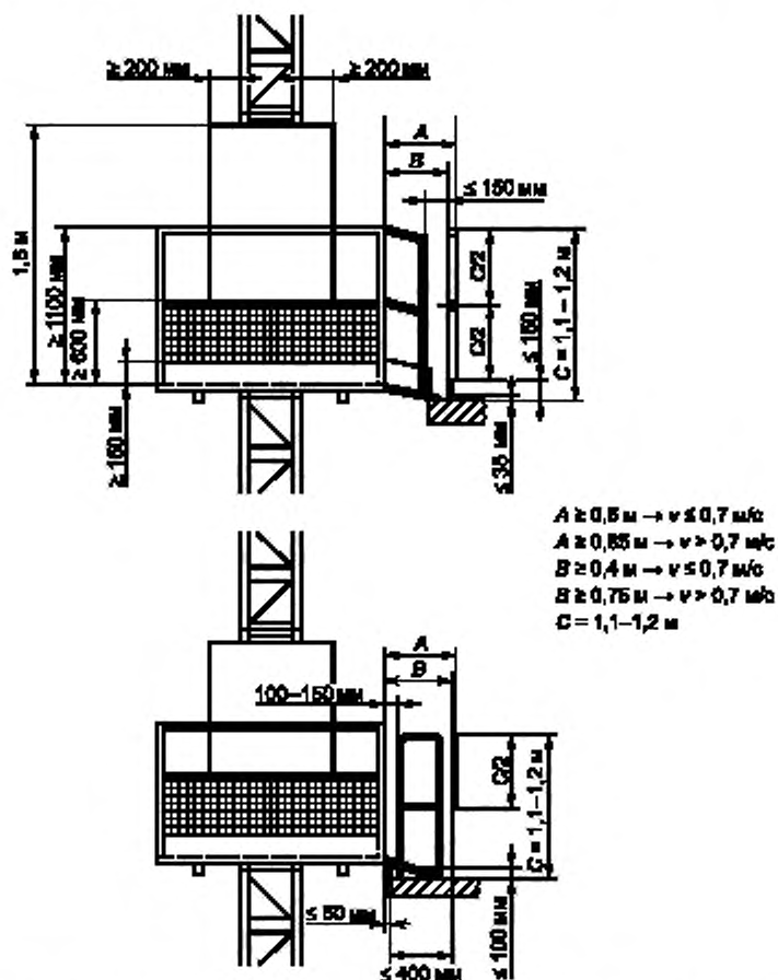
Рисунок 6 — Пример дверей погрузочной площадки уменьшенной высоты
