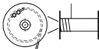
Рисунок 13 — Способы заделки концов проволочного каната
