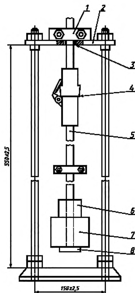
1 — анкерное крепление гибкого кабеля; 2 — монтажная плита; 3 — втулка; 4 — соединитель электроприбора; 5 — гибкий кабель; 6 — дополнительный груз; 7 — основной груз; 8 — фланец несущего устройства
