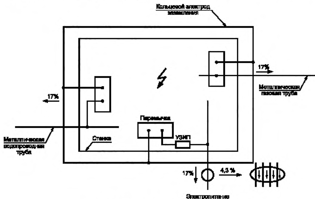
Рисунок А.1 — Общее распределение грозового тока
