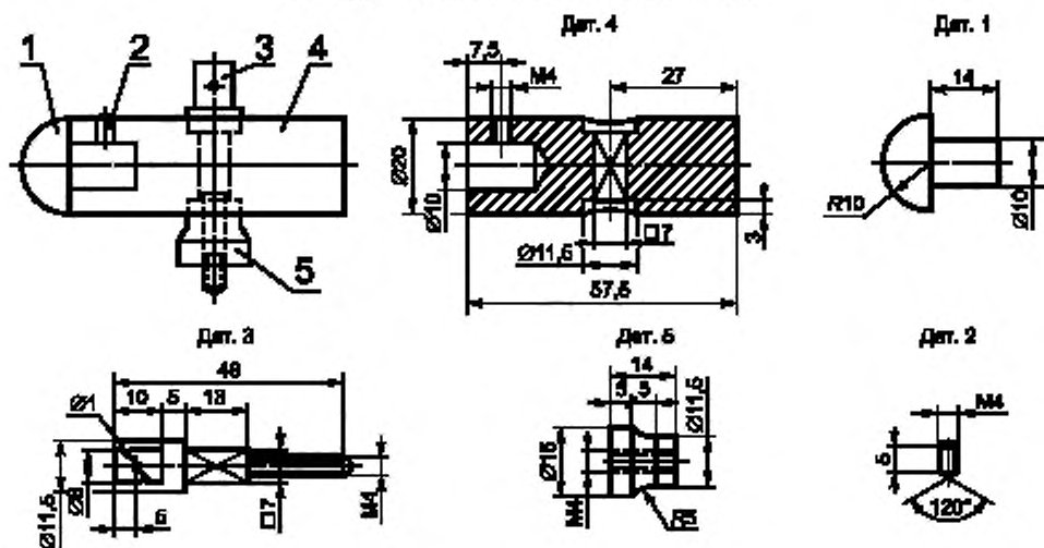
b — Ударный элемент маятникового молотка
