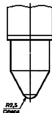
Рисунок 12б — Нагрузочный стержень для испытания давлением шарика
