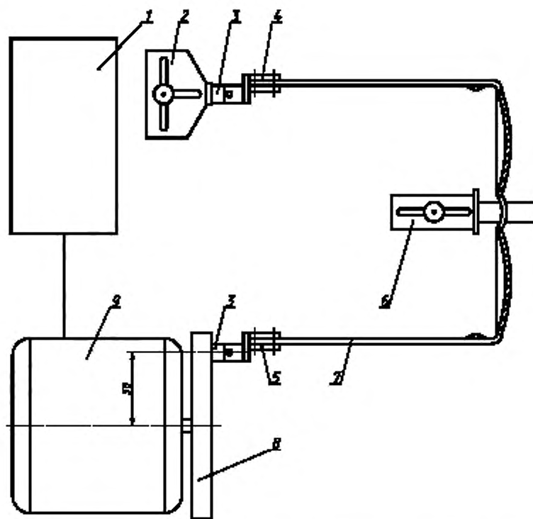
1 — контрольная панель и счетчик; 2 — регулятор зажима заушика; 3 — универсальный шарнир; 4 — фиксированный зажим R ; 5 — подвижный зажим M ; 6 — узел поддержки моста; 7 — испытуемый образец; 8 — вращающийся диск; 9 — приводной мотор
