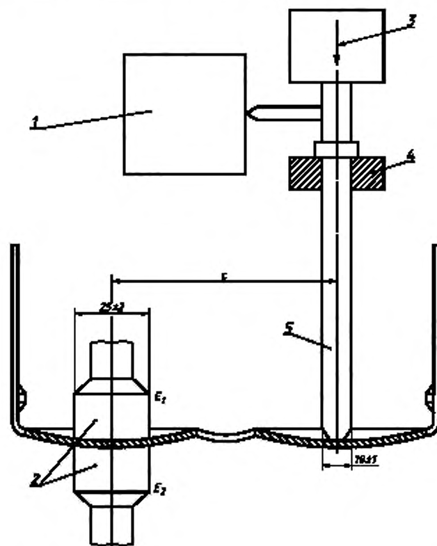
1 — измерительный прибор; 2 — кольцевая струбцина; 3 — направление и точка приложения силы (наибольшая — 5 Н); 4 — направляющее кольцо; 5 — давящий штырь; E_1 и E_2 — контактные поверхности
