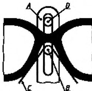
А — вертикальная стойка с щелью для регулирования по высоте; В — горизонтальный стержень, пропущенный через щель в вертикальной стойке А и закрепленный стопорным устройством для фиксации выбранной высоты; С — жесткая металлическая пластина, согнутая через горизонтальный стержень В, вращающаяся вокруг стержня при перемещении очковой оправы; D — ограничительный стержень, пропущенный через прорезь вертикальной стойки А и закрепленный стопорным устройством для фиксации выбранной высоты
