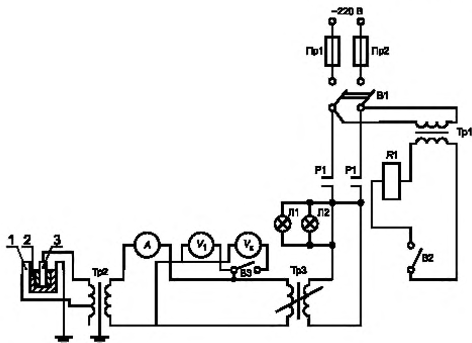
A — амперметр с ценой деления от 0 до 10 А; B1 — двухполюсный выключатель на 220 В; B2 , B3 — однополюсные выключатели; L1 , L2 — сигнальные лампы; V1 — рабочий вольтметр от 0 до 110 В; V2 — контрольный вольтметр от 0 до 110 В; Pr1 , Pr2 — плавкие предохранители; P1 — магнитный пускатель; Tr1 — трансформатор на 220/24 В; Tr2 — трансформатор 60000/110 В мощностью 2,0 кВ · А; Tr3 — регулирующий трансформатор от 0 до 110 В; 1 — ванна; 2 — корпус моноблока; 3 — электрод
