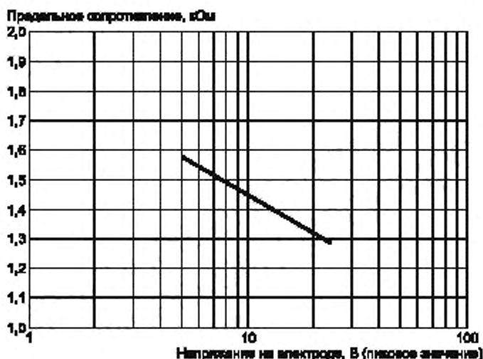
Рисунок 101 — Кривая предельного сопротивления для оглушающего оборудования
