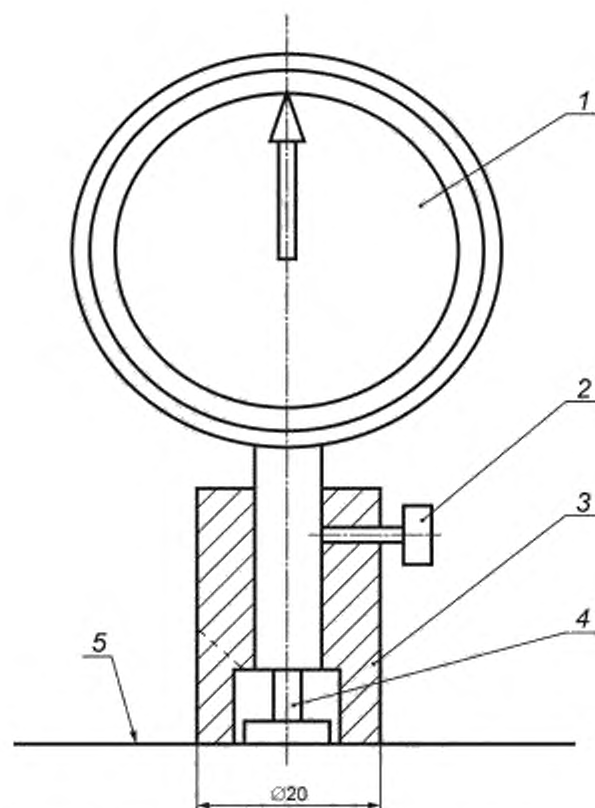
1 — индикатор; 2 — столбовый винт; 3 — ограничительная оправка; 4 — наконечник индикатора — фланец; 5 — торцевая плоскость оправки 3 и фланца 4 индикатора
