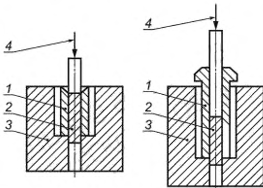
1 — корпус шипа; 2 — износостойкий элемент; 3 — подставка; 4 — направление выдавливания
