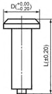
Рисунок 2 — Рекомендуемые размеры шипа с предельно допустимыми отклонениями
