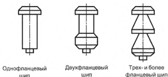
Рисунок 1 — Виды шипов по количеству фланцев
