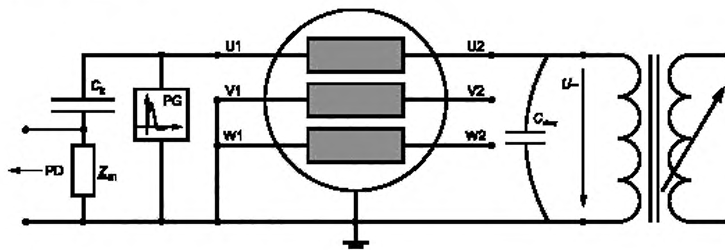
Рисунок 7 — Нормализация измерительной цепи для соединений S1.1
