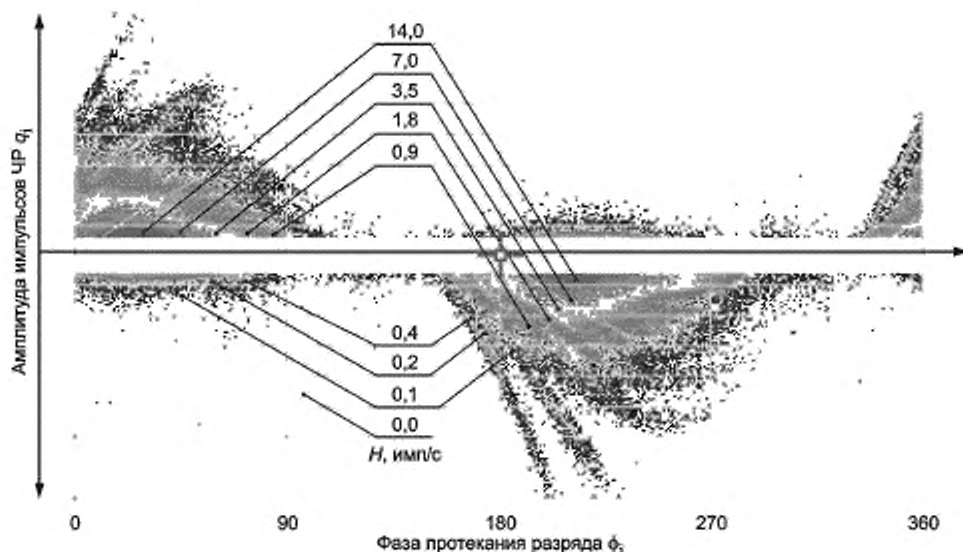
Рисунок 4 — Пример \varphi - q - л диаграммы рассеяния импульсов ЧР на объекте, представленном на рисунке 5б.
