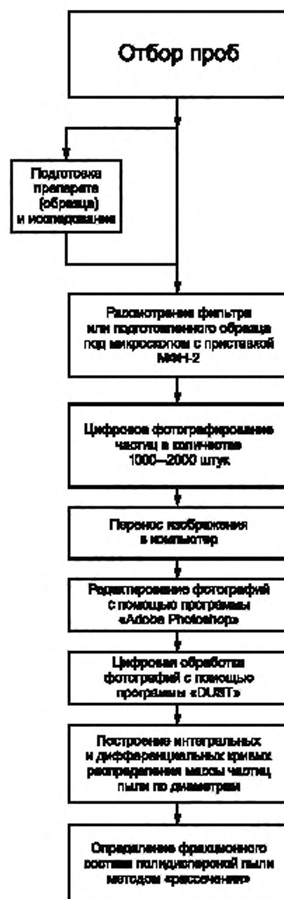
Рисунок 1 — Блок-схема методики микроскопического анализа
