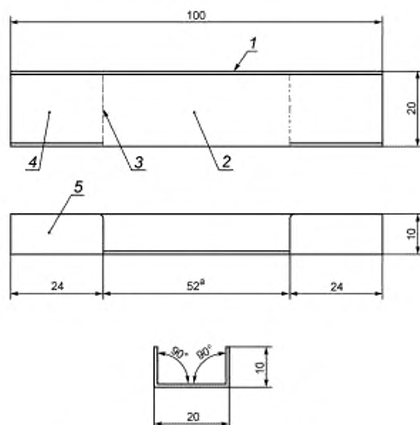
а) Металлический лоток для выравнивания образца
