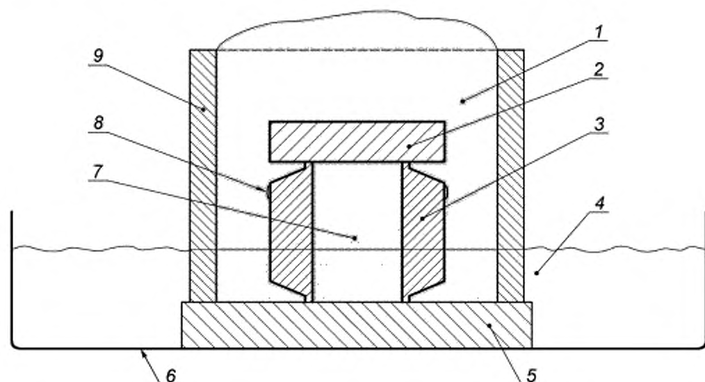
1 — дублиционный материал на основе агара; 2 — пластина, образующая верхнюю поверхность; 3 — форма для изготовления образца; 4 — вода для охлаждения; 5 — стеклянная пластина; 6 — контейнер с охлаждающей водой; 7 — образец; 8 — резиновая лента (размерами приблизительно 0,8 × 5 мм); 9 — полимерная кольцевая опока
