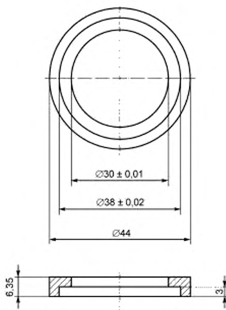
б) фиксатор кольцевой формы б
