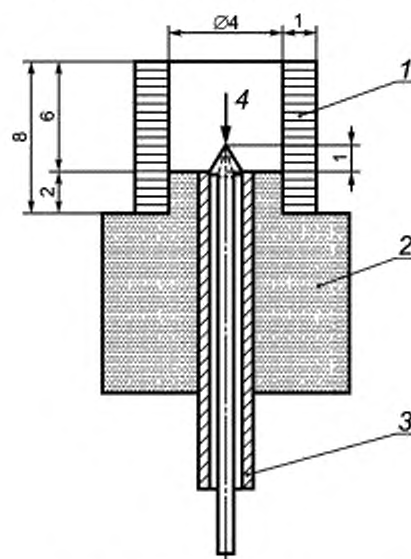
1 — полиэтиленовая трубка; 2 — полиамидный блок; 3 — трубка из нержавеющей стали, 4 — коническая вершина спая термопары
