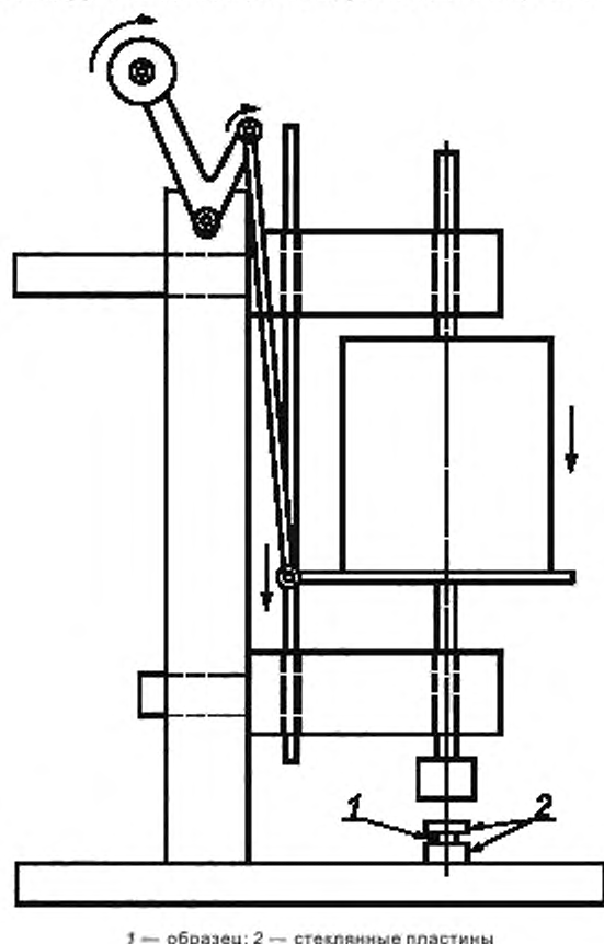
Рисунок 1 — Нагружающее устройство
