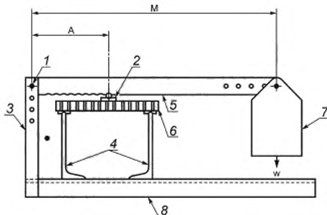
1 — точка поворота; 2 — опора рычага; 3 — основание рычага; 4 — опора образца; 5 — плечо нагрузки; 6 — образец; 7 — ящик для груза; 8 — основание; M — расстояние между точкой поворота и точкой приложения веса, A — расстояние между точкой поворота и точкой приложения силы; W — вес плеча нагрузки
