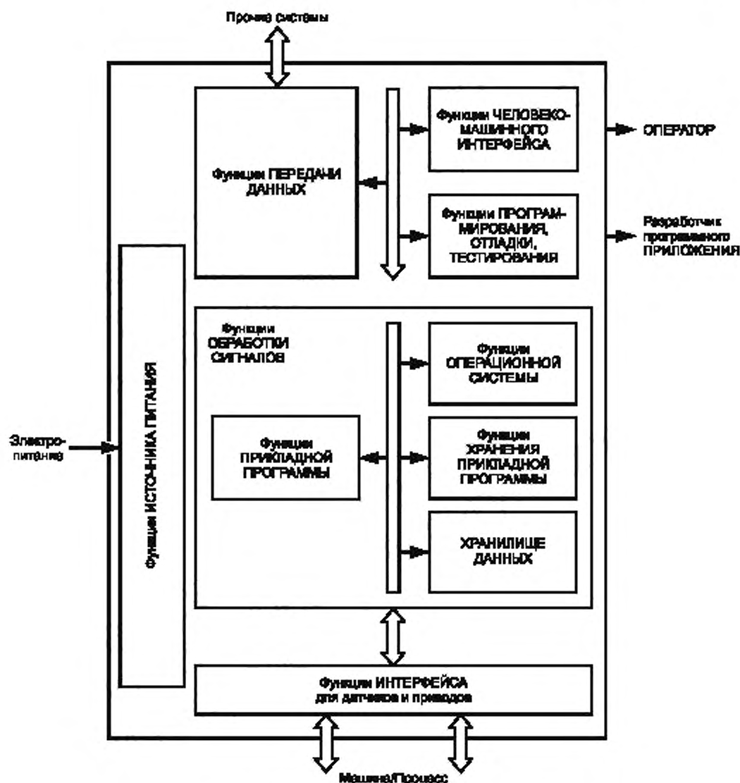
Рисунок 1 — Базовая функциональная структура ПЛК-системы
