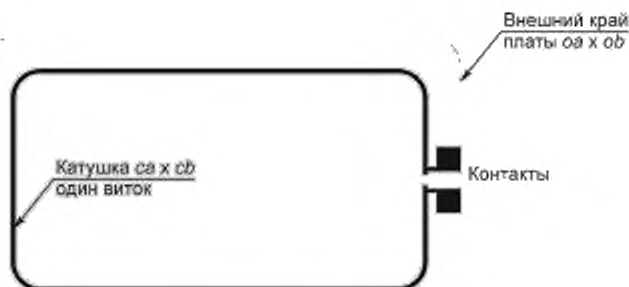
Рисунок 1 — Пример калибровочной катушки
