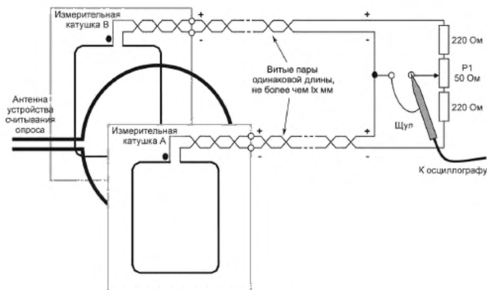
Рисунок 6 — Пример испытательной установки
