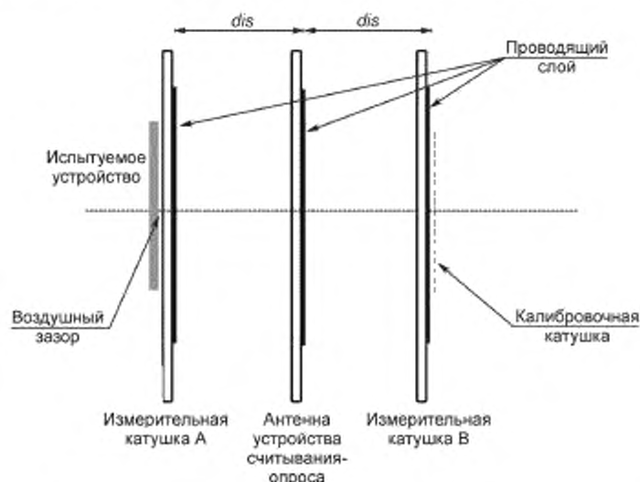
Рисунок 3 — Комплект испытательного устройства считывания/опроса
