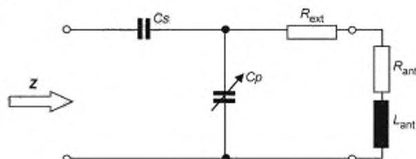
Рисунок В.1 — Схема согласования импеданса
