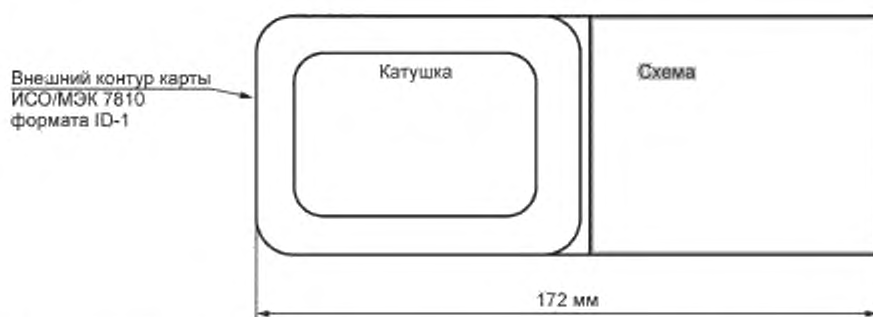
Рисунок 4 — Пример эталонной радиочастотной метки, соответствующей размеру идентификационной карты согласно требованиям ИСО
