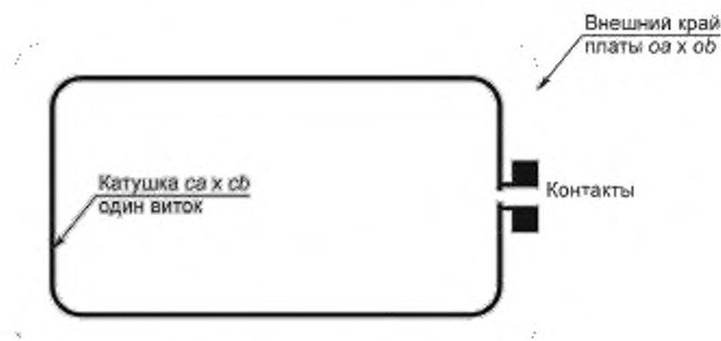
Рисунок 5 — Пример калибровочной катушки
