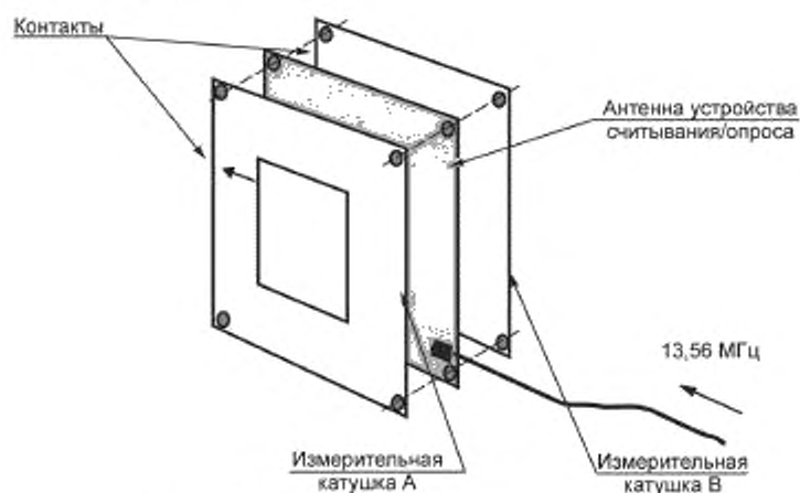
Рисунок Е.2 — Комплект измерительной катушки
