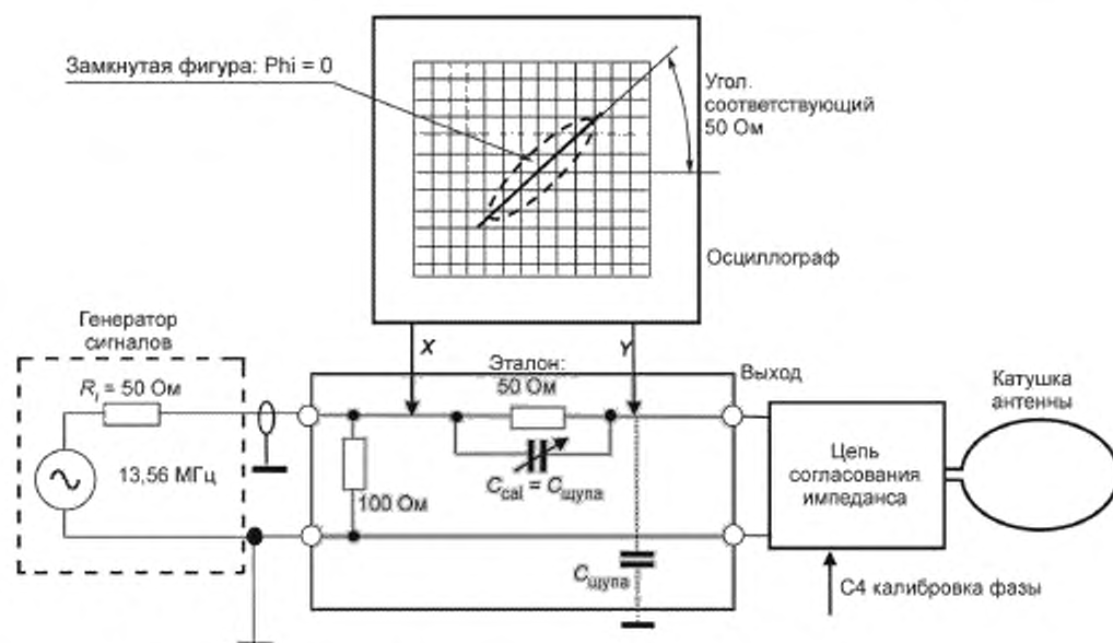
Рисунок D.2 — Предустановки при калибровке (этап 2)
