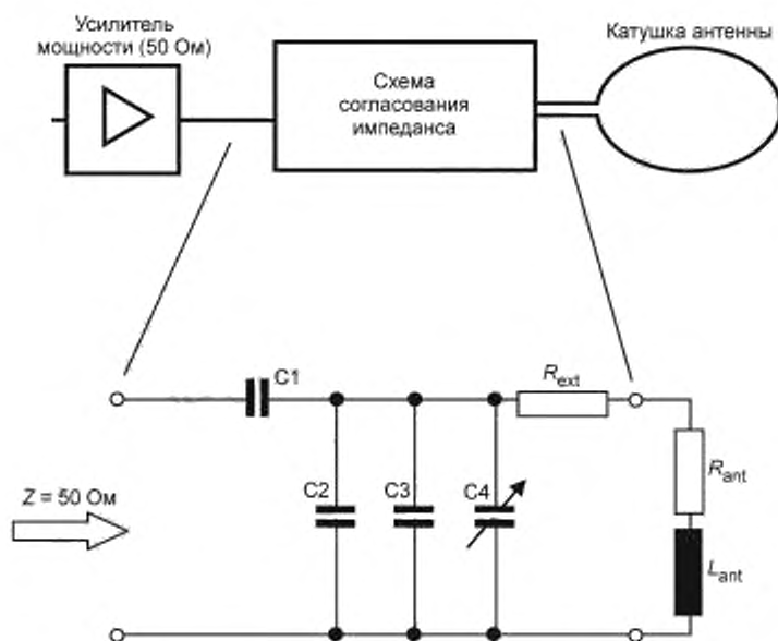
Рисунок С.3 — Схема согласования импеданса
