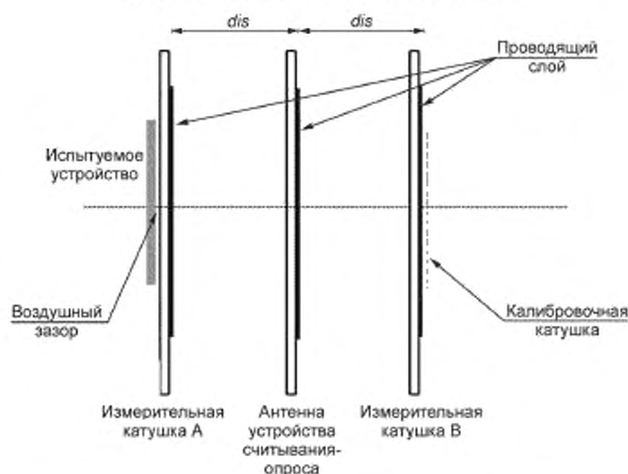
Рисунок 7 — Комплект испытательного устройства считывания/опроса
