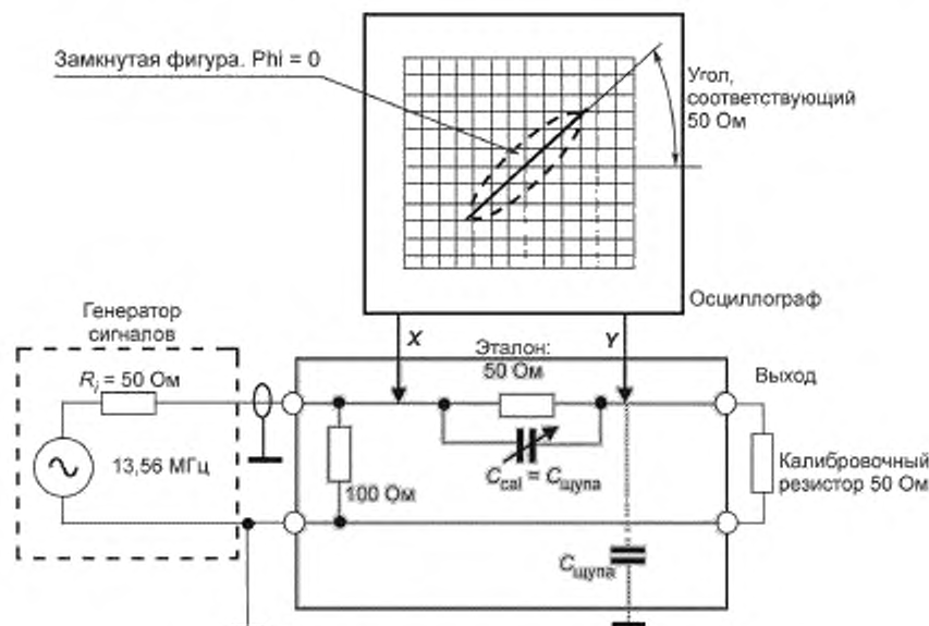
Рисунок D.1 — Предустановки при калибровке (этап 1)
