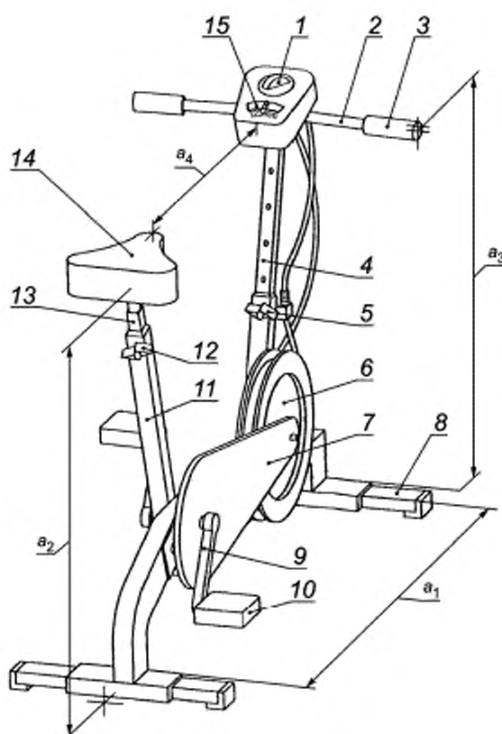
1 — регулятор нагрузки; 2 — руль; 3 — рукоятка; 4 — вынос руля; 5 — регулятор высоты руля; 6 — маховик; 7 — кожух; 8 — рама; 9 — колесо педали; 10 — педаль; 11 — подседельная труба рамы; 12 — регулятор высоты сиденья; 13 — стойка сиденья; 14 — сиденье; 15 — дисплей значений мощностей; a_1 — a_4 — размеры, измеряемые при испытаниях несущей способности
