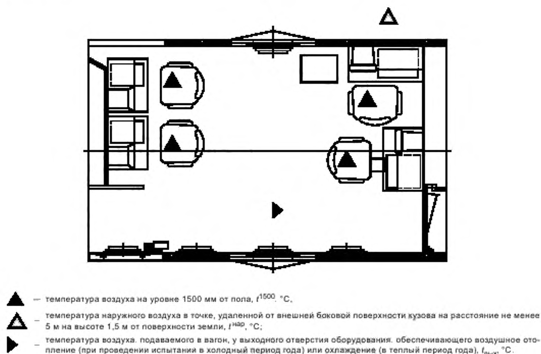
Рисунок И.5 — Размещение точек измерения параметров при проведении испытаний по определению показателей эффективности системы обеспечения микроклимата в операторской СПС
