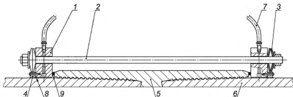
1 — металлический фланец; 2 — шпилька; 3 — пружины; 4 — гайка; 5 — муфта; 6 — ниппельный элемент; 7 — гибкий шланг; 8 — уплотнительное кольцо; 9 — плоская прокладка
