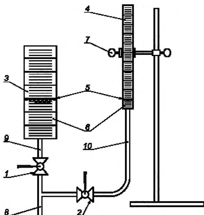
1 — вентиль перед большим градуированным цилиндром; 2 — вентиль перед небольшим градуированным цилиндром; 3 — большой открытый сверху градуированный цилиндр на 100–200 см 3 ; 4 — небольшой открытый сверху градуированный цилиндр примерно на 25 см 3 с ценой деления 0,1 см 3 ; 5 — уровень воды; 6 — подкрашенная вода; 7 — регулируемый держатель, позволяющий в начале каждого периода выдержки разместить дно цилиндра на уровне, соответствующем от 100 до 200 см 3 ; 8 — гибкий шланг, соединенный с верхней частью камеры при испытании внутренним давлением газа и с верхним отверстием одной из торцевых заглушек при испытании внешним давлением; 9 — гибкий шланг к большому цилиндру; 10 — гибкий шланг к небольшому цилиндру
